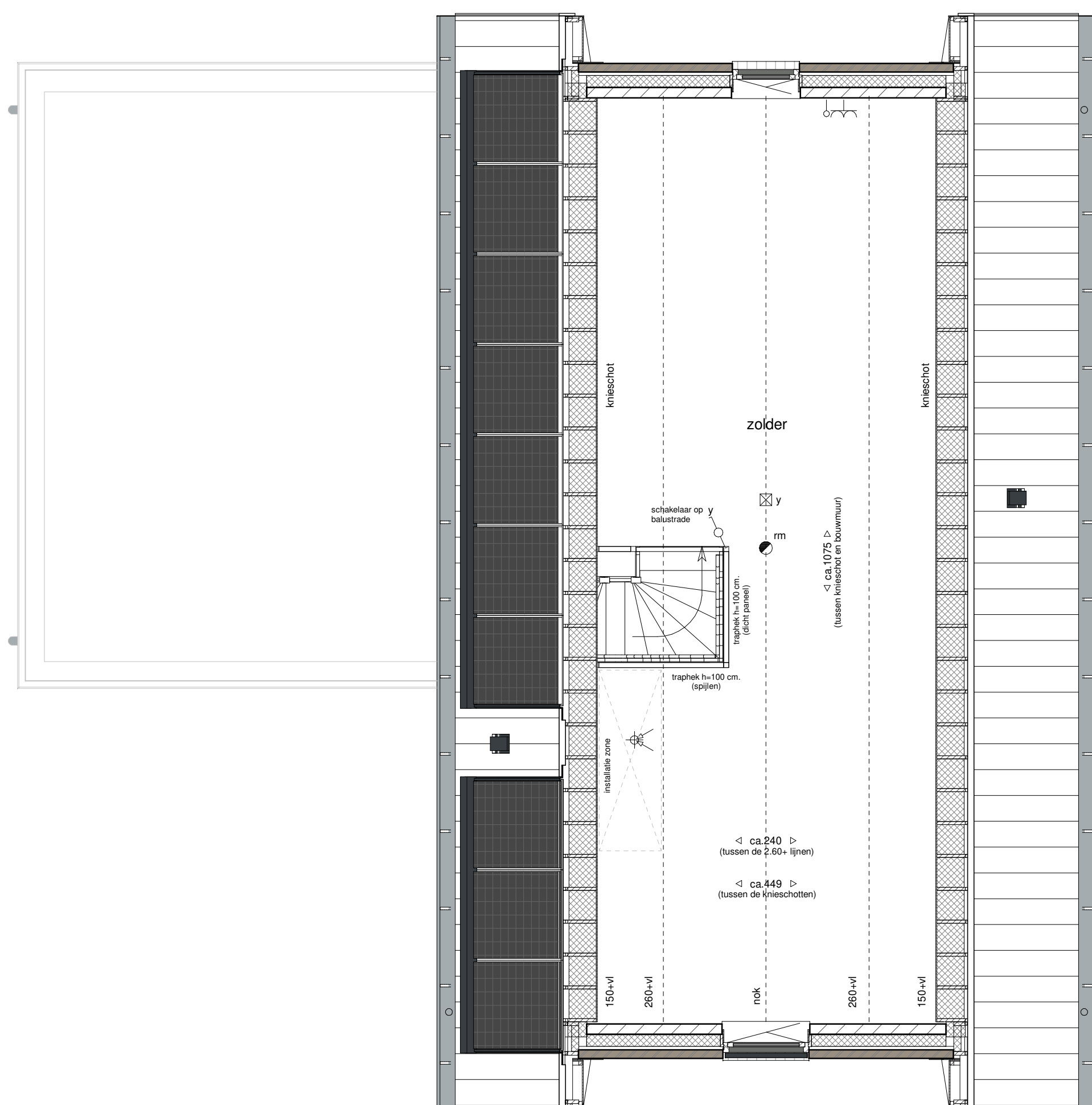
tweede verdieping 1 : 50
