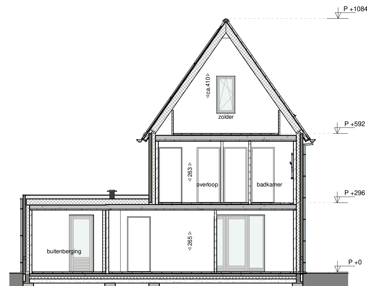
dwarsdoorsnede 1 : 100
