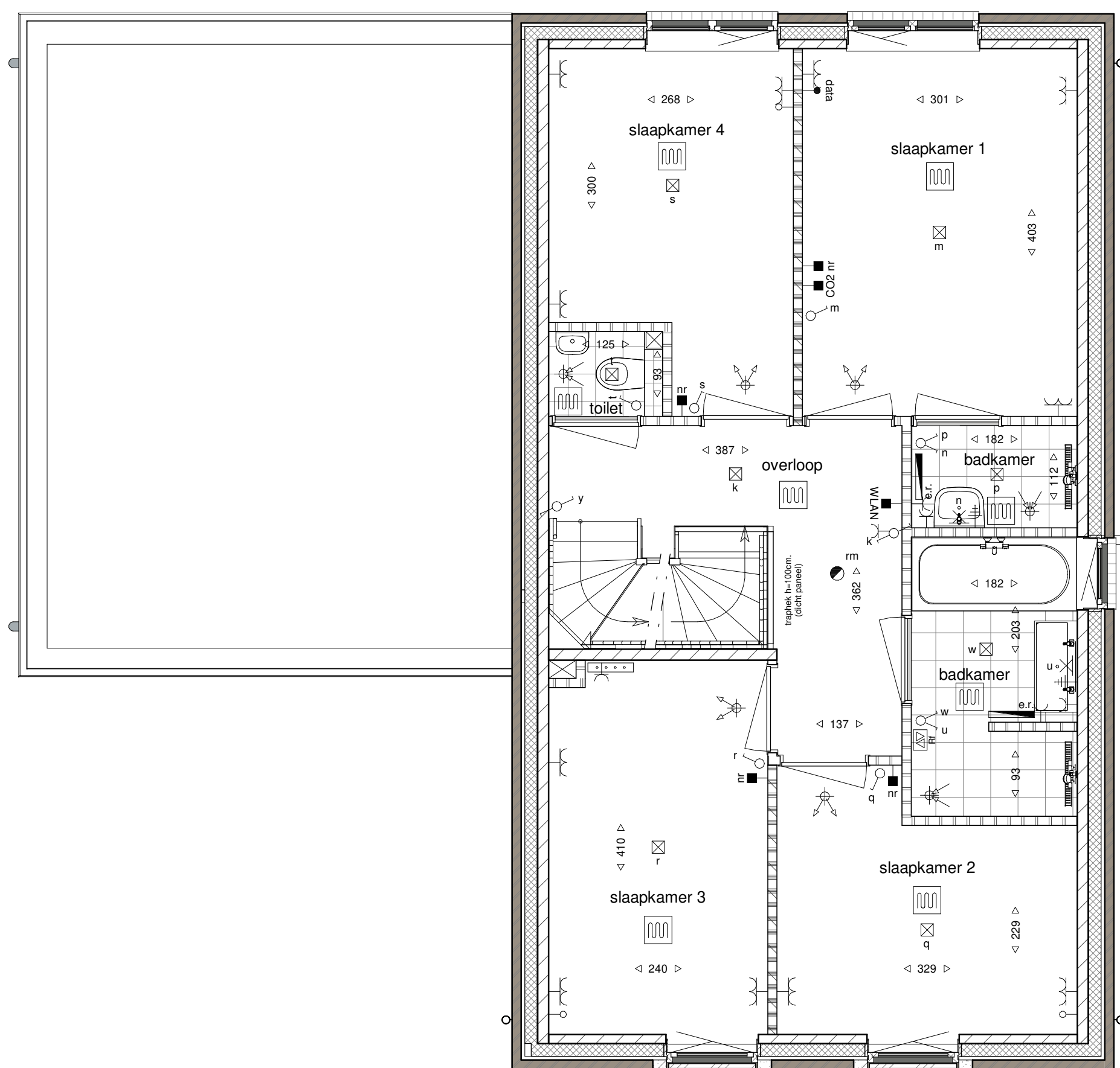
eerste verdieping 1 : 50
