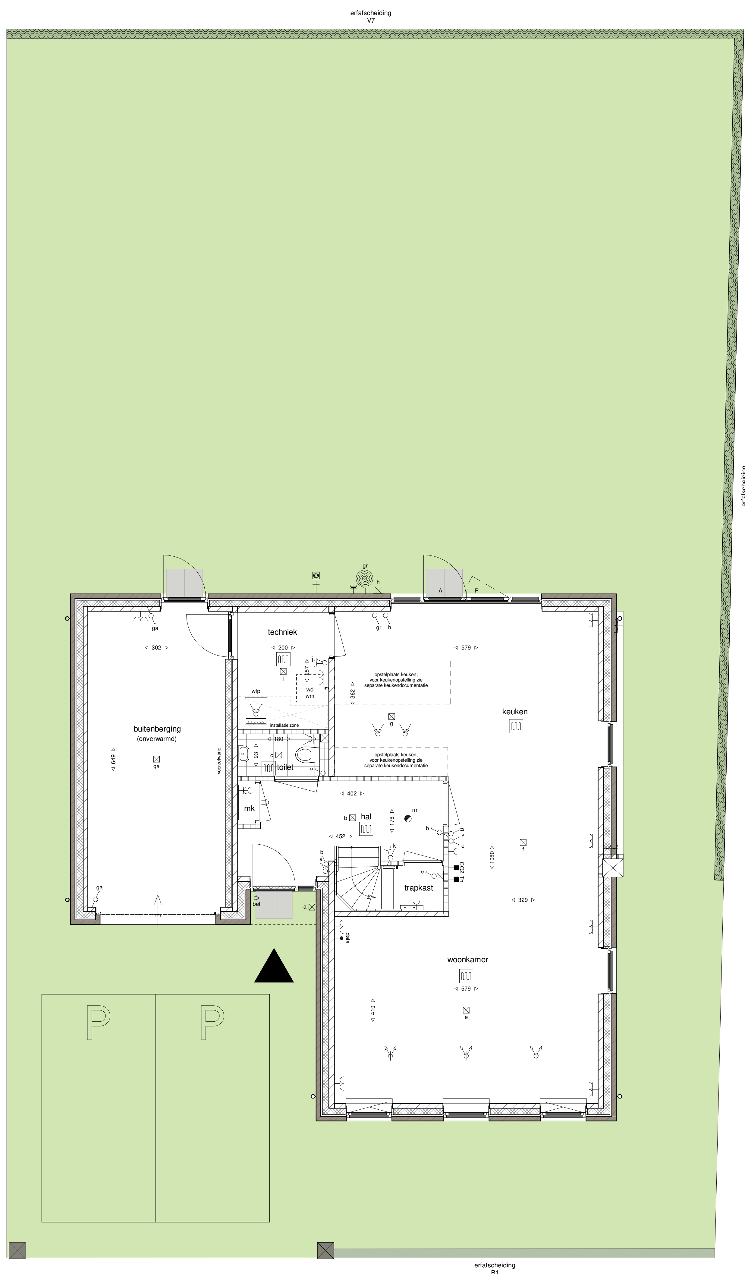
begane grond 1 : 50
