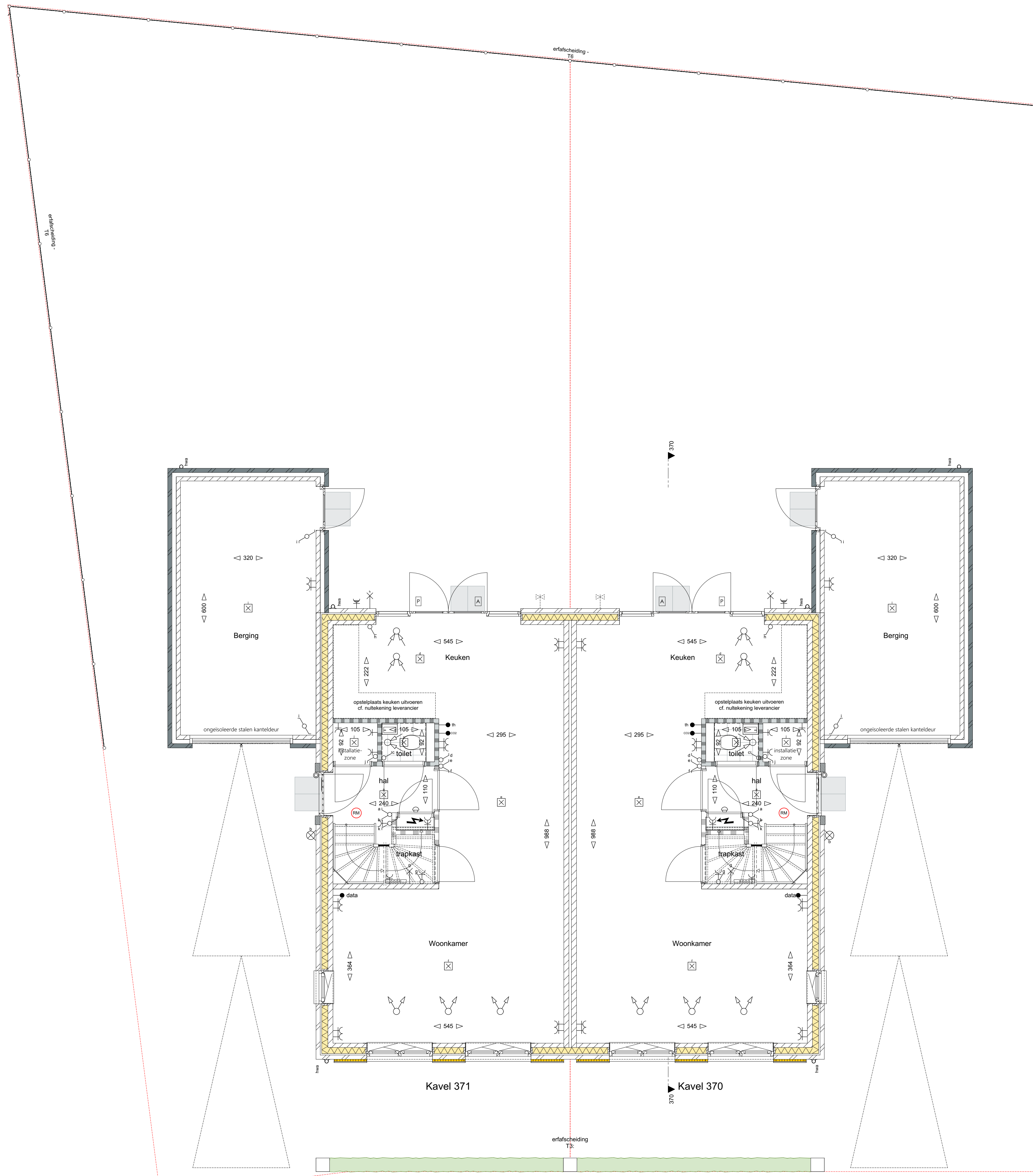
Begane grond
