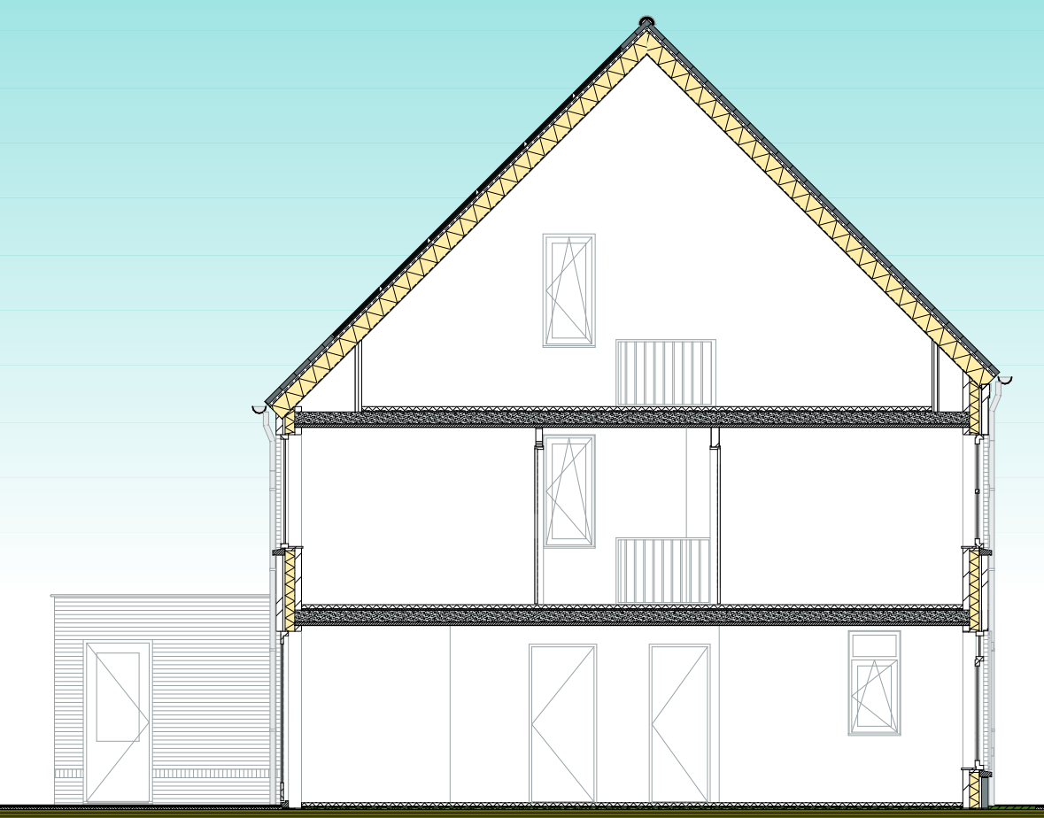
Doorsnede 370
