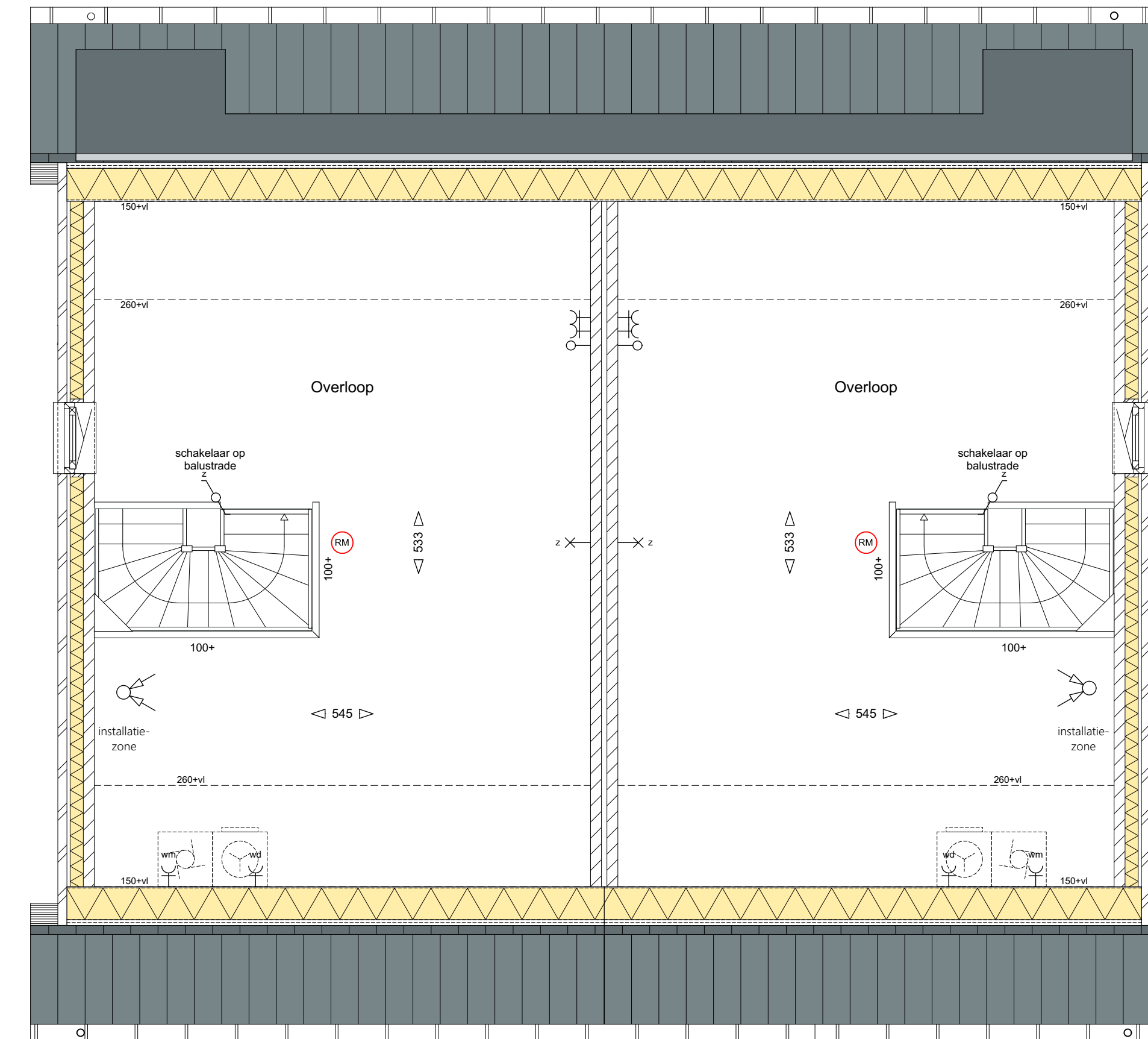
2e verdieping
