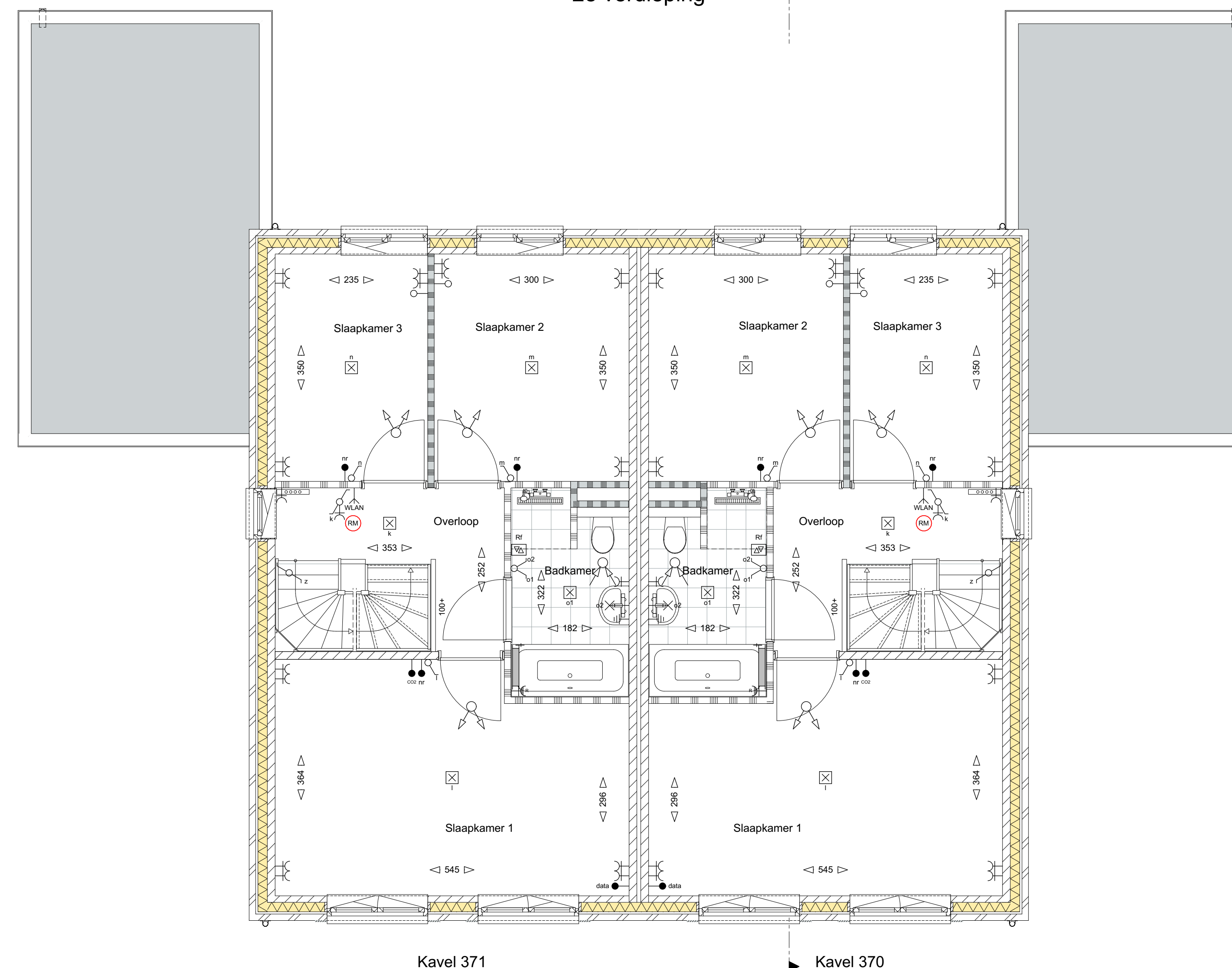
2e verdieping
