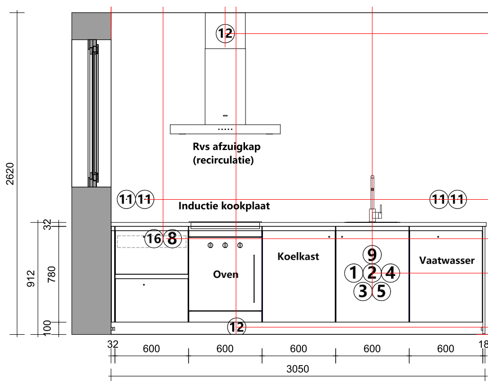
Vooraanzicht
