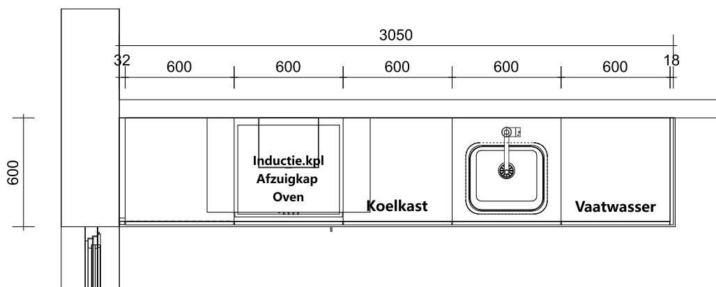
Plattegrond
