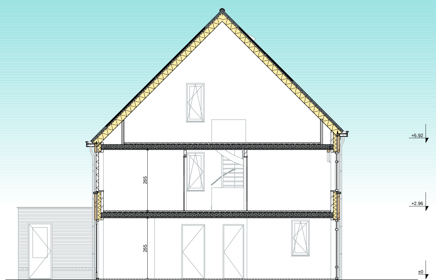
Doorsnede 107
