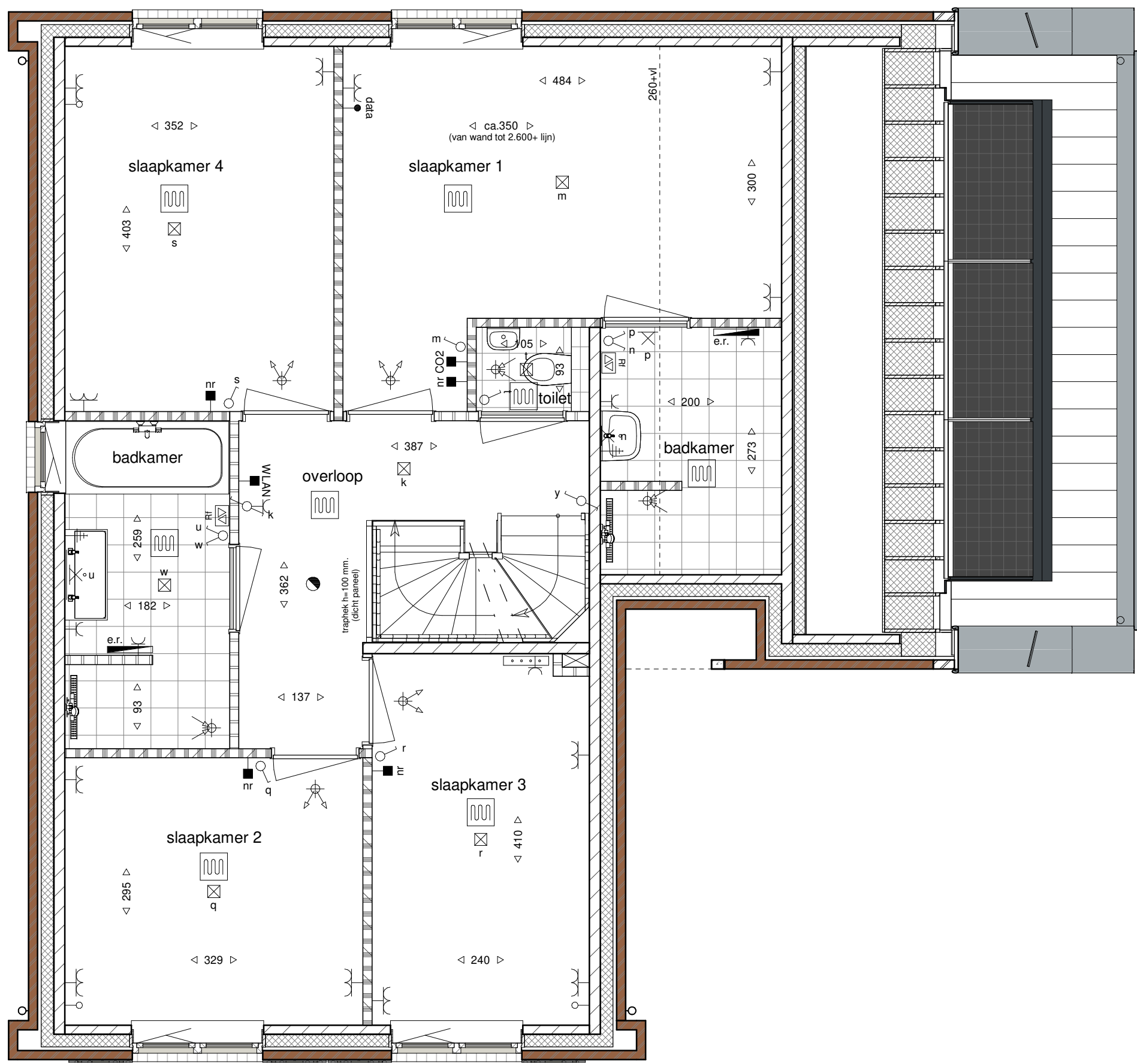
eerste verdieping 1 : 50
