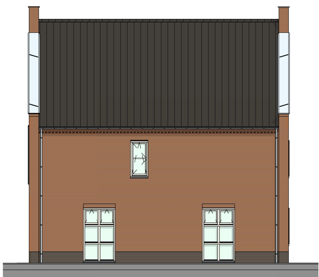
zijgevel links 1 : 100
