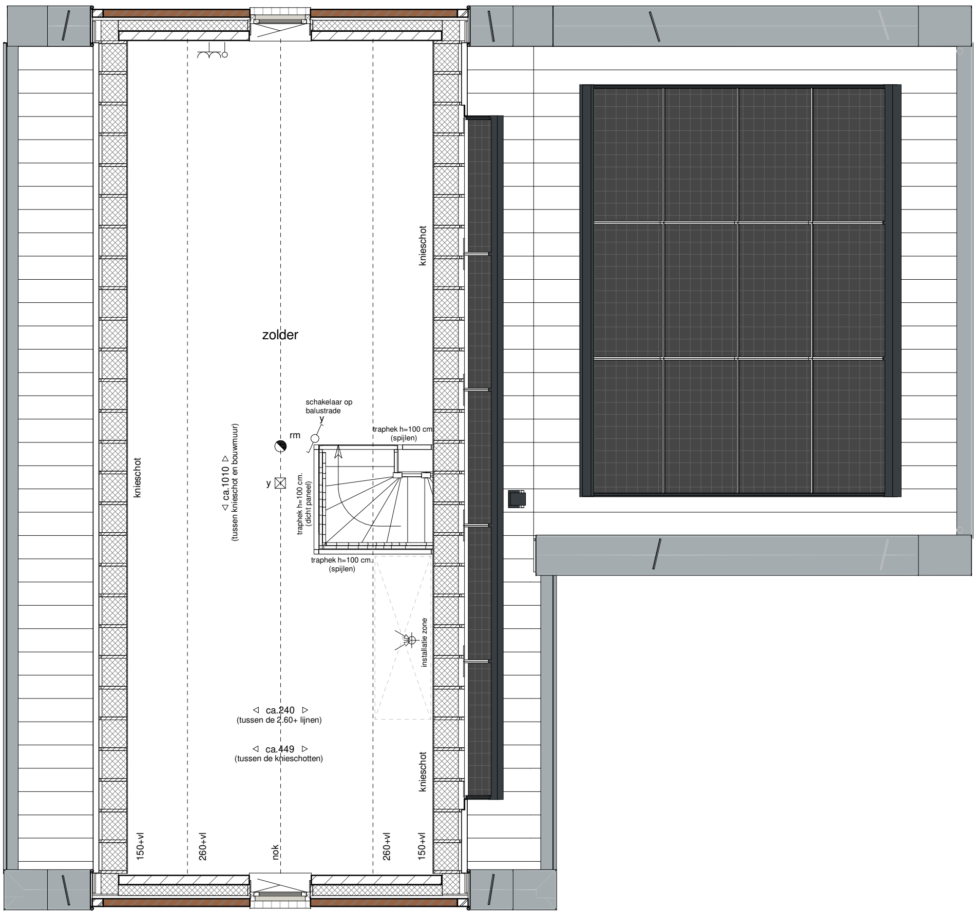
tweede verdieping 1 : 50
