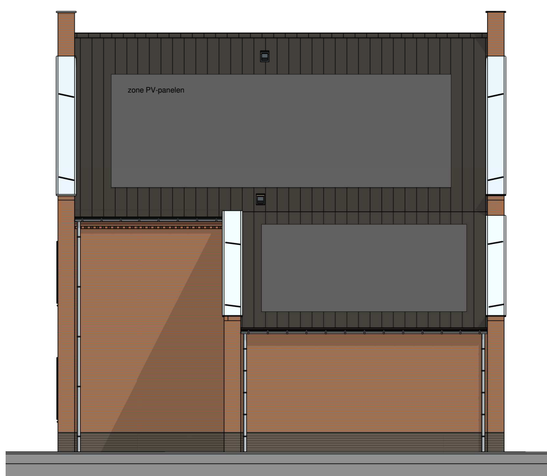
zijgevel rechts 1 : 100
