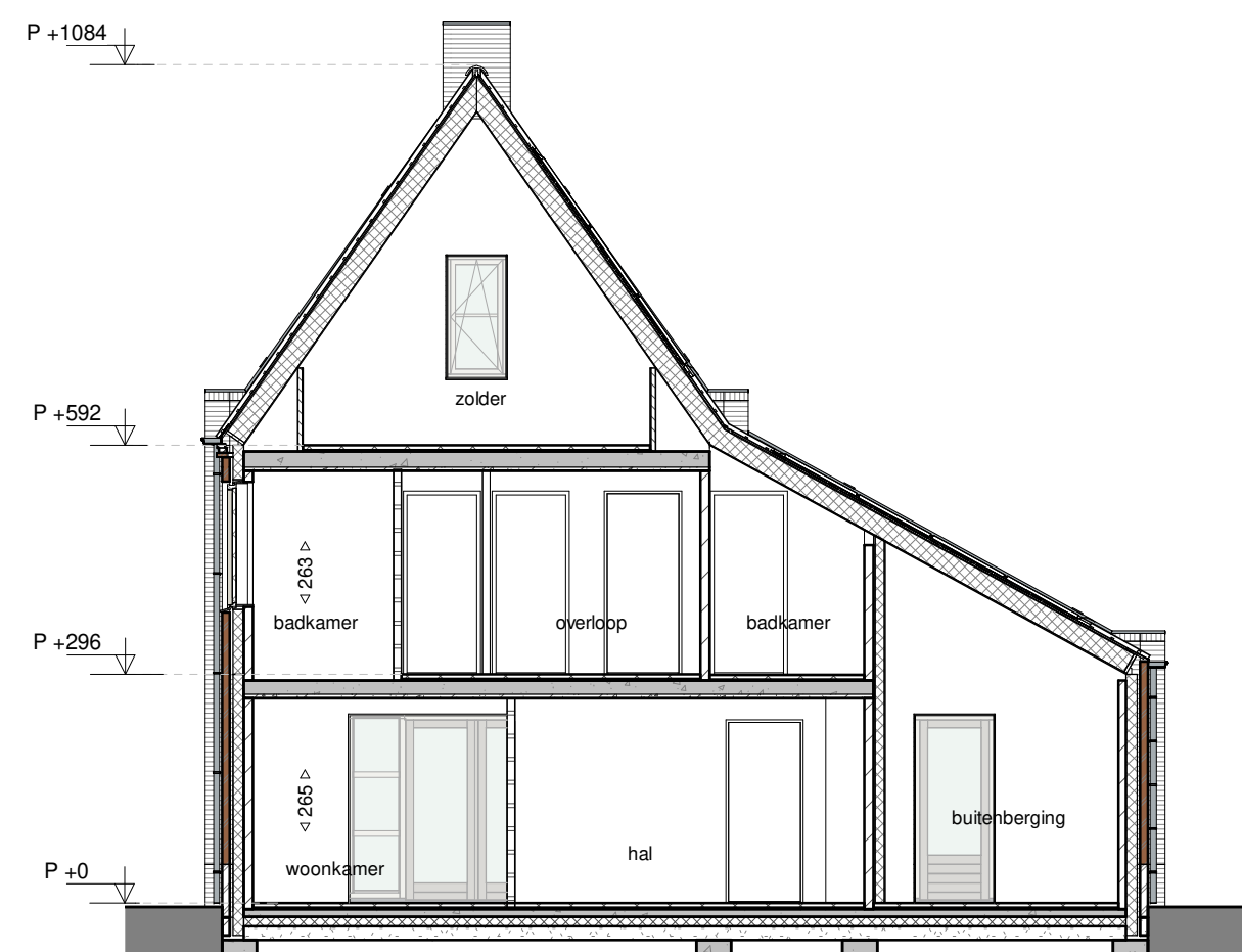
dwarsdoorsnede 1 : 100
