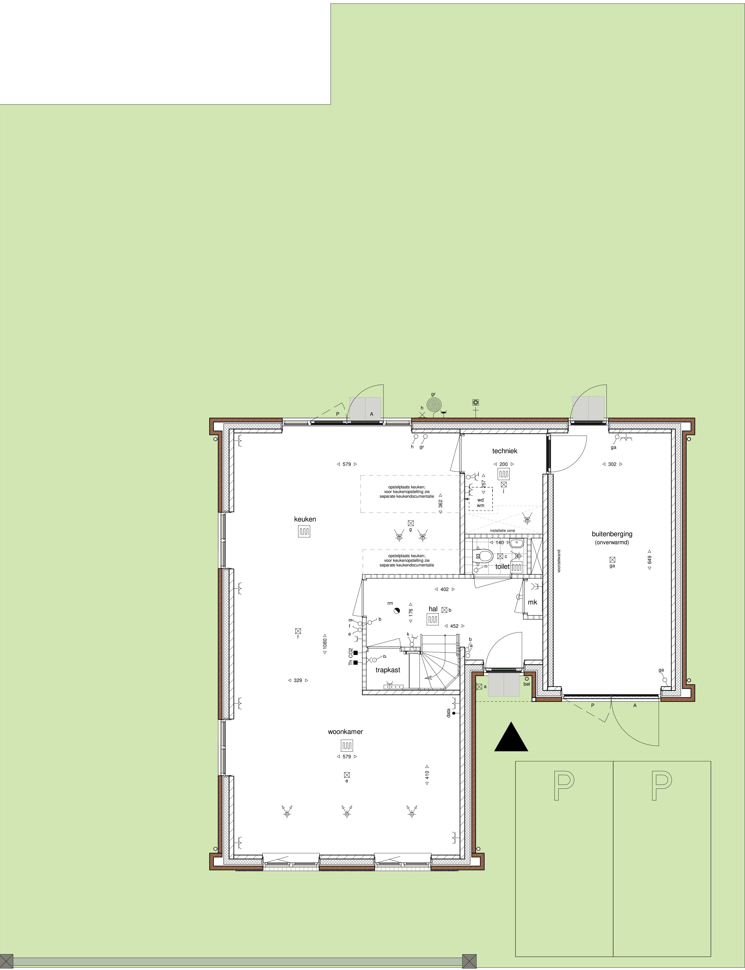
begane grond 1 : 50
