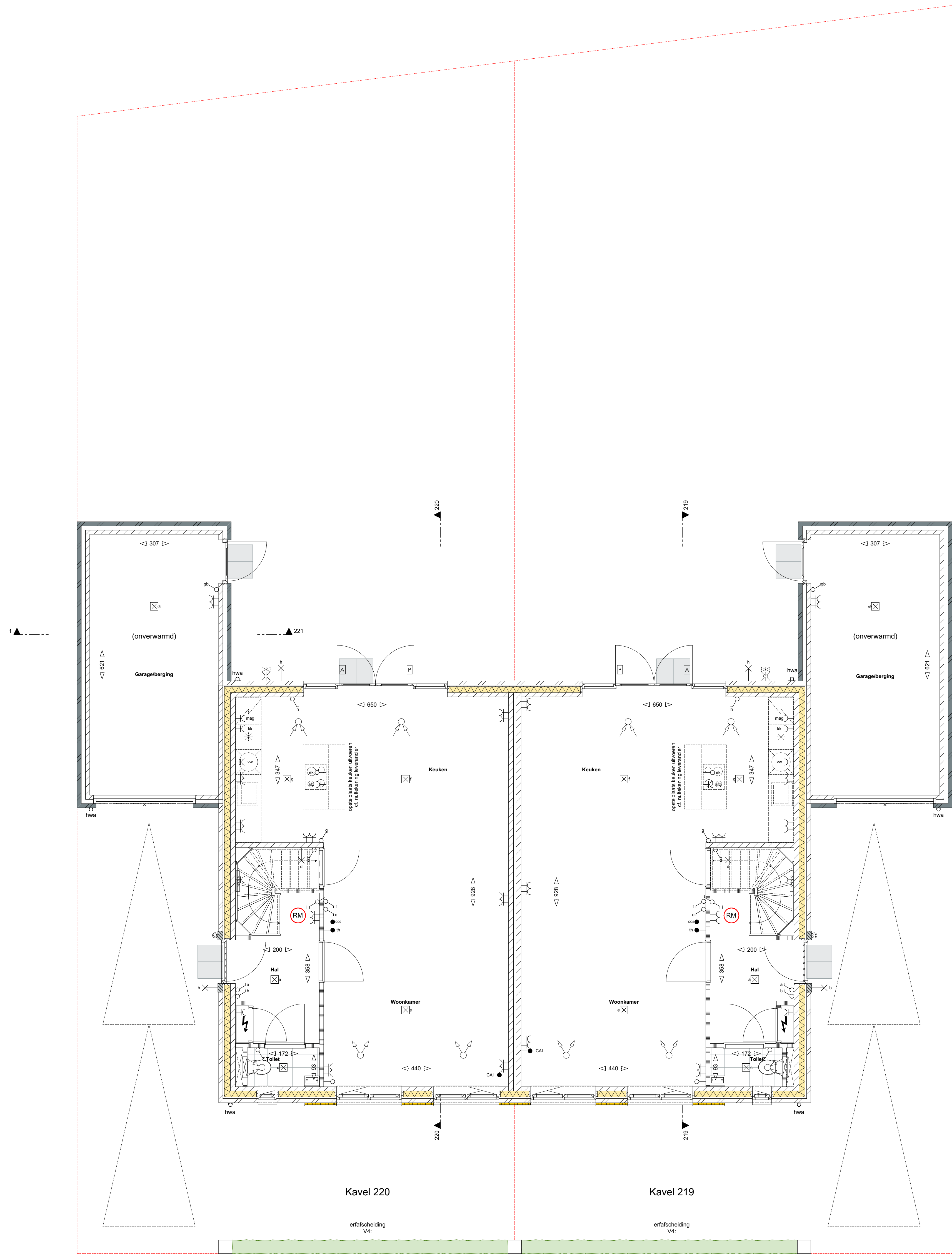
Begane grond
