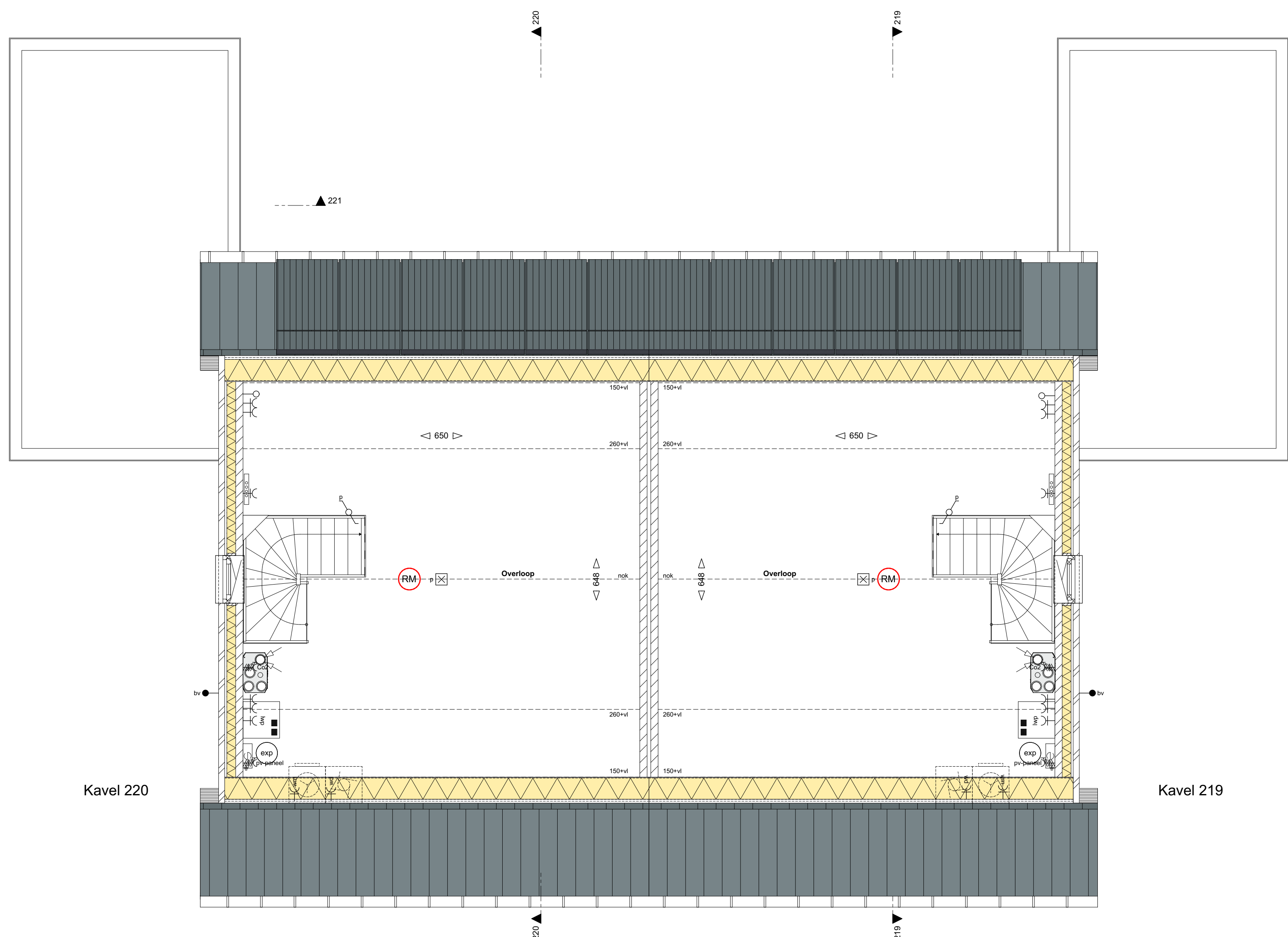
2e verdieping
