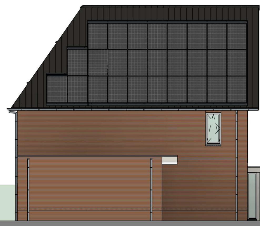
Linkergevel
