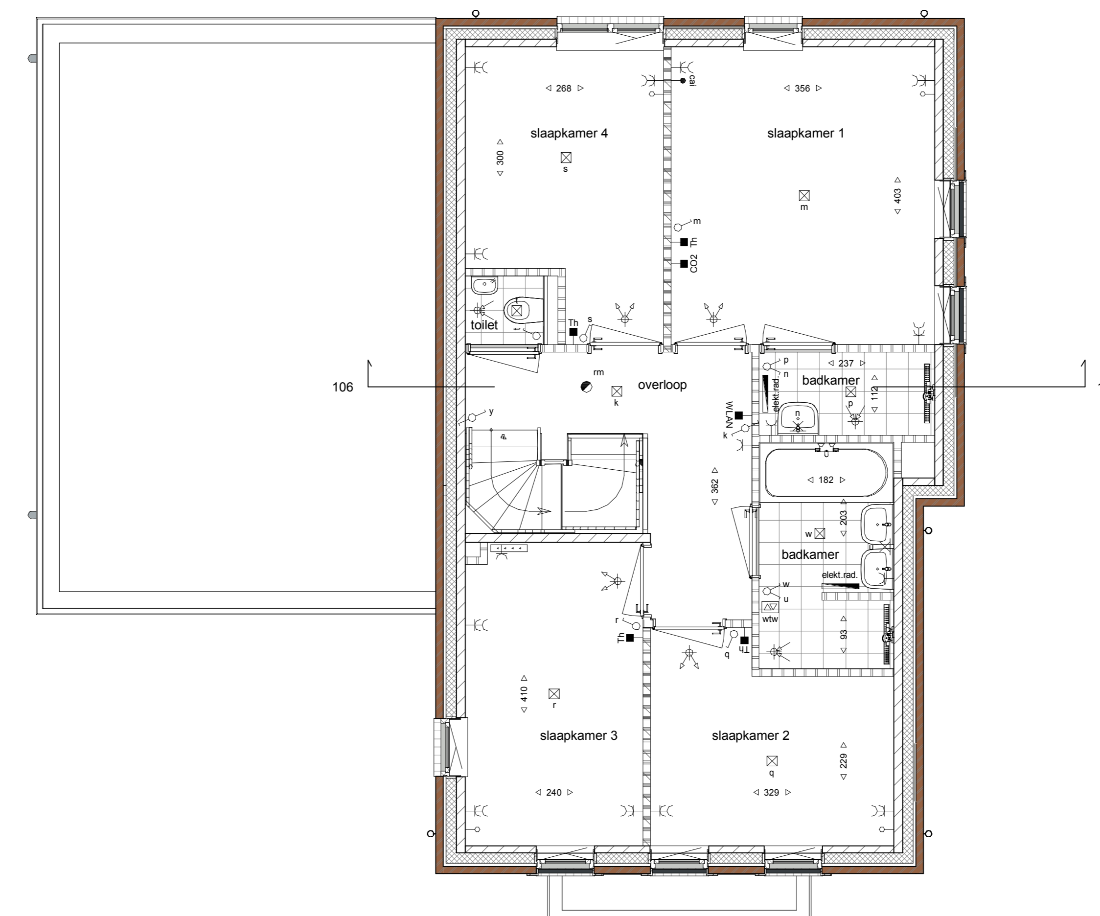
1e verdieping
