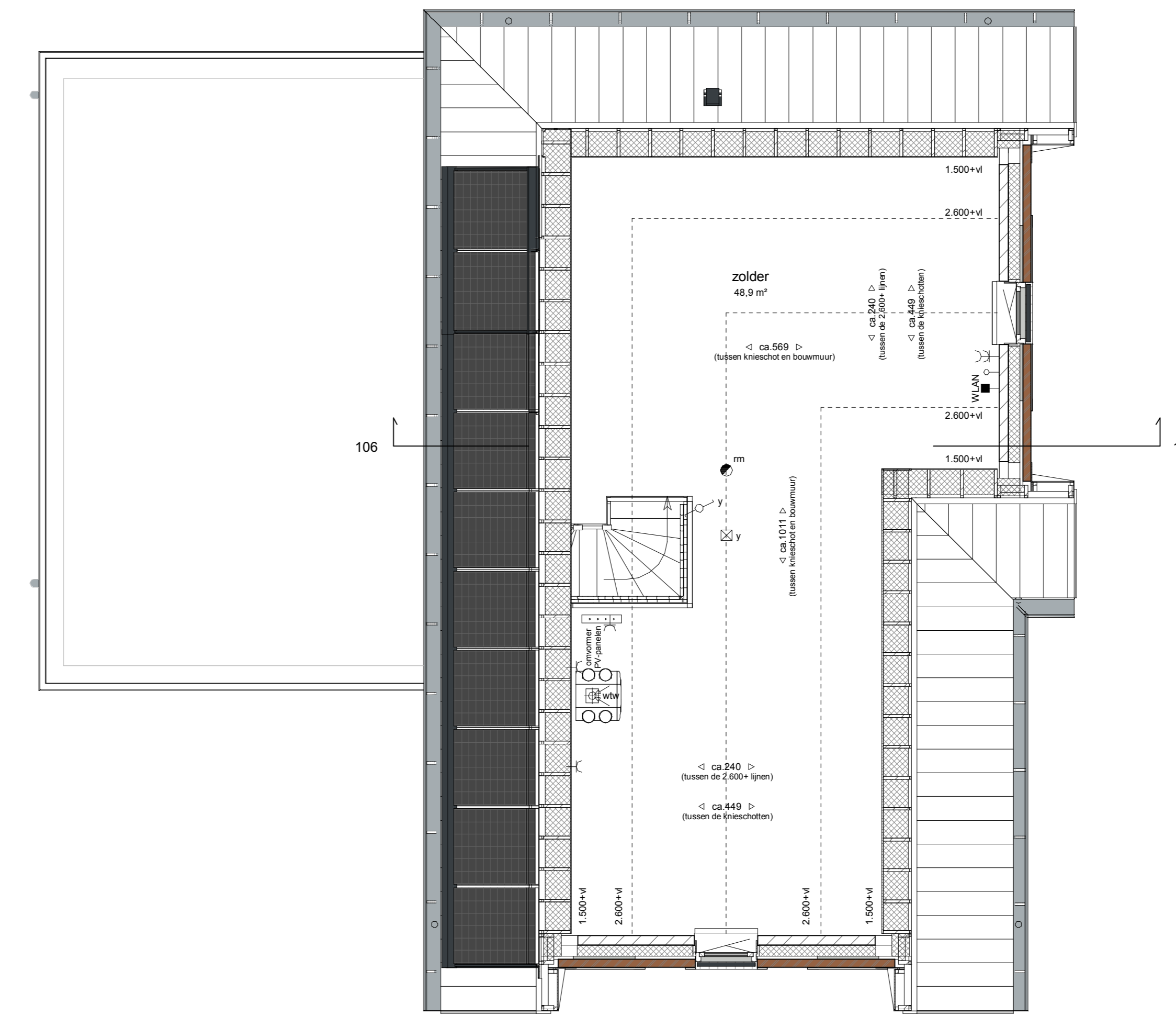
2e verdieping
