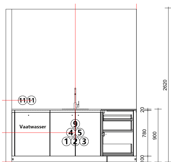
Vooraanzichten
