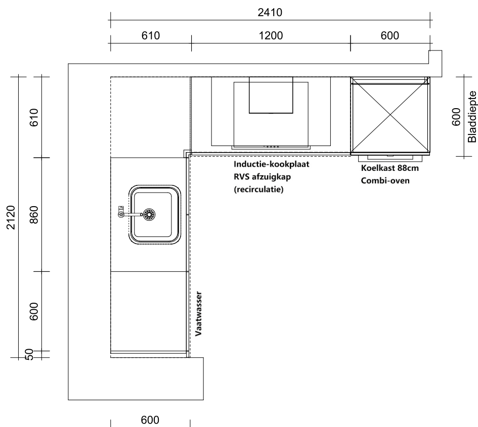
Plattegrond
