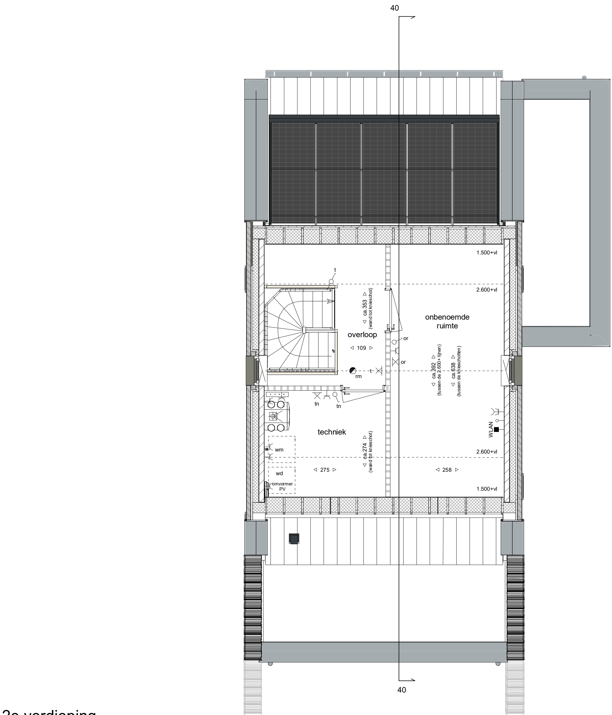
2e verdieping
