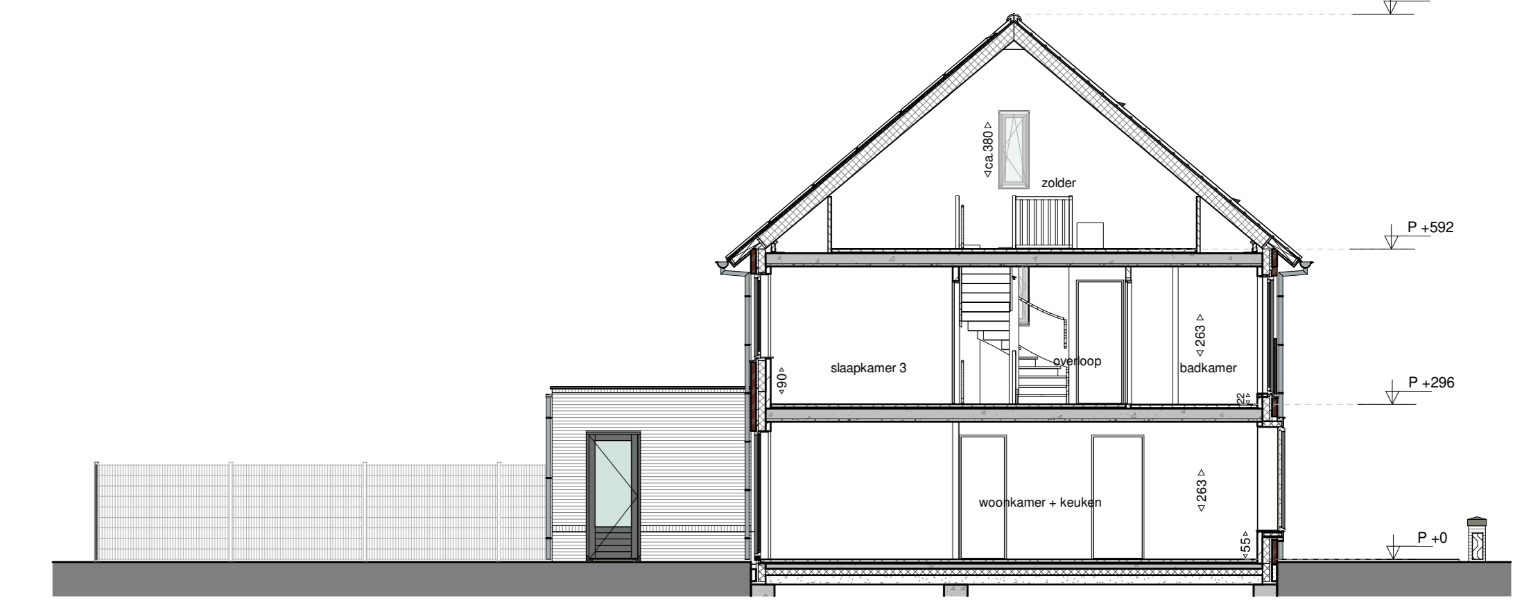
dwarsdoorsnede 1 : 100
