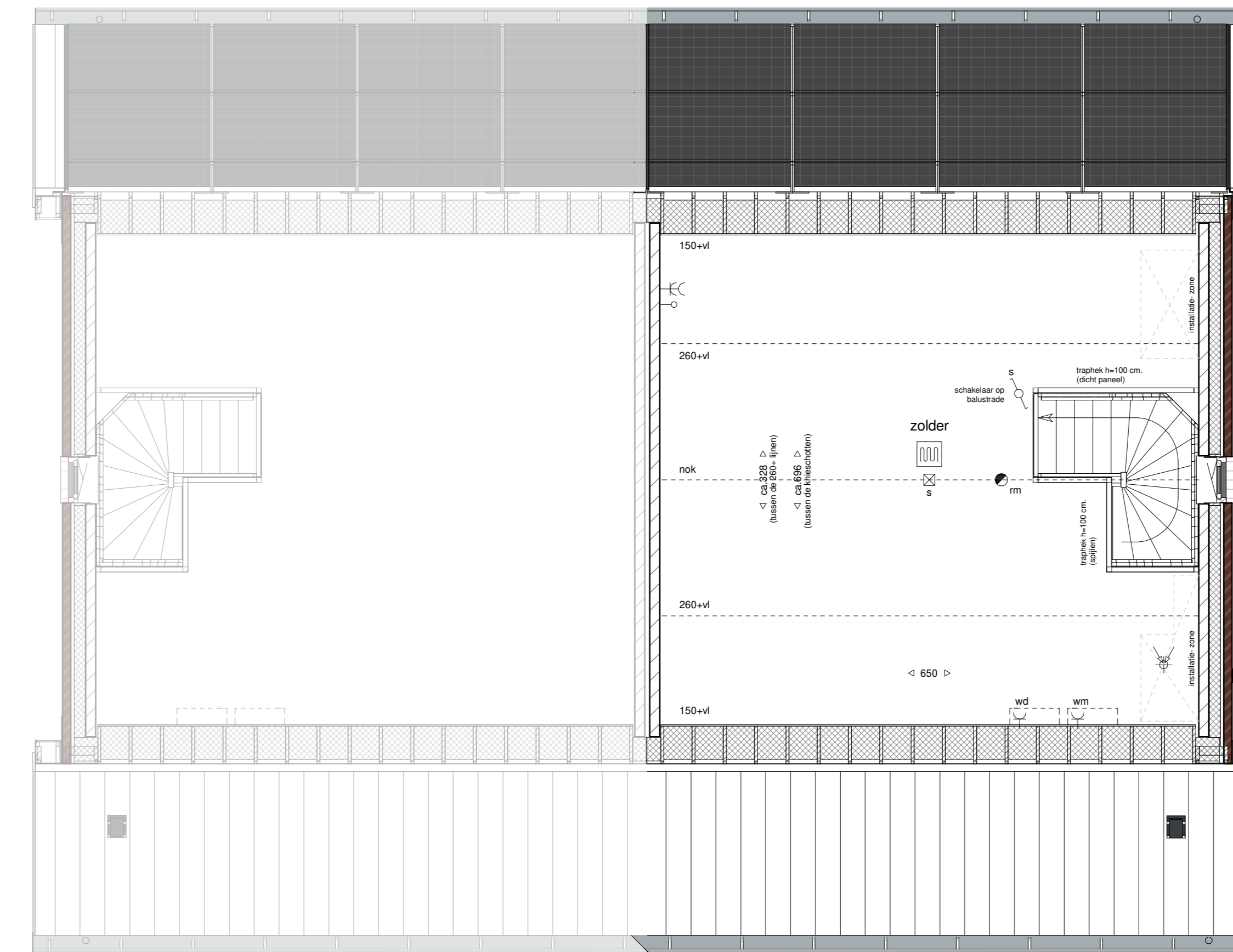
tweede verdieping 1 : 50
