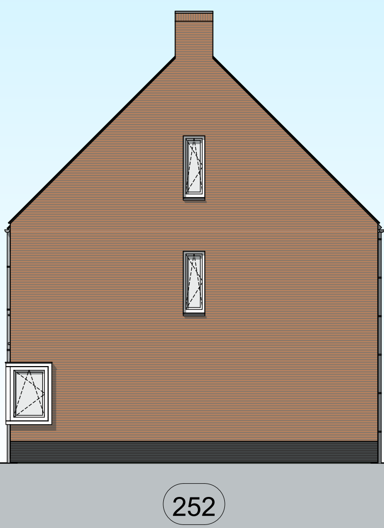
RECHTER ZIJGEVEL
