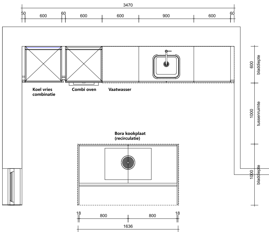
Plattegrond
