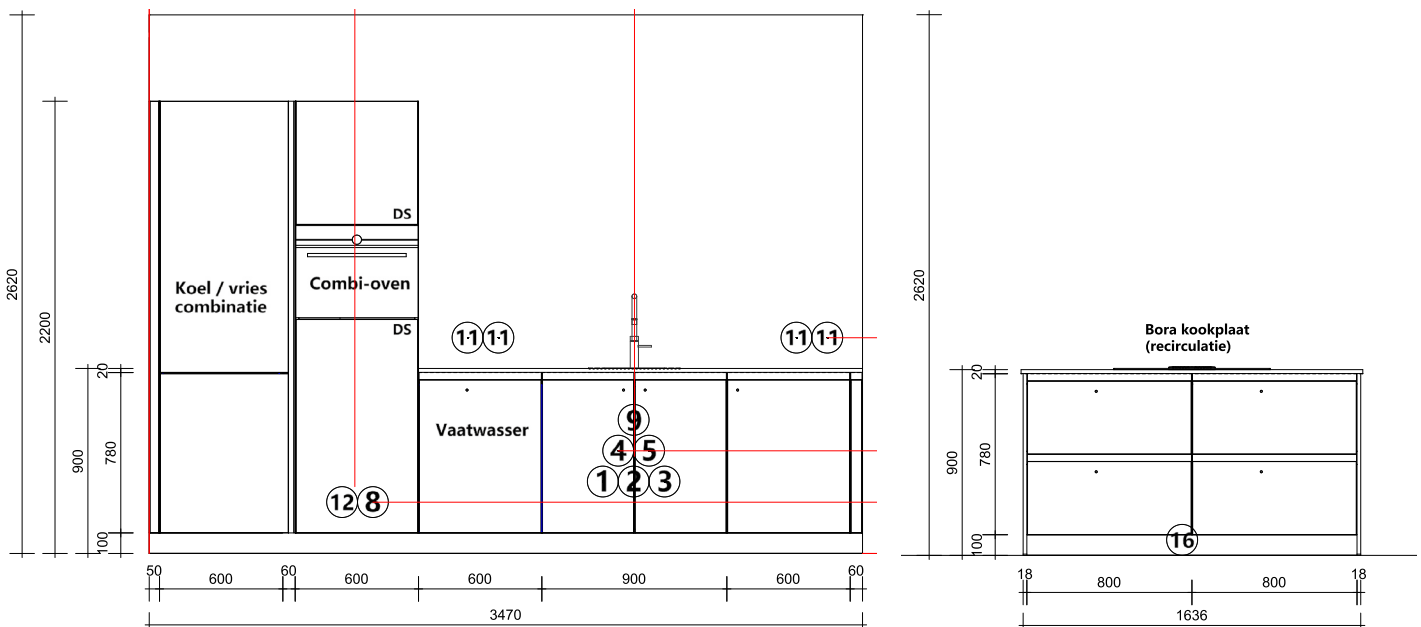
Vooranzichten
