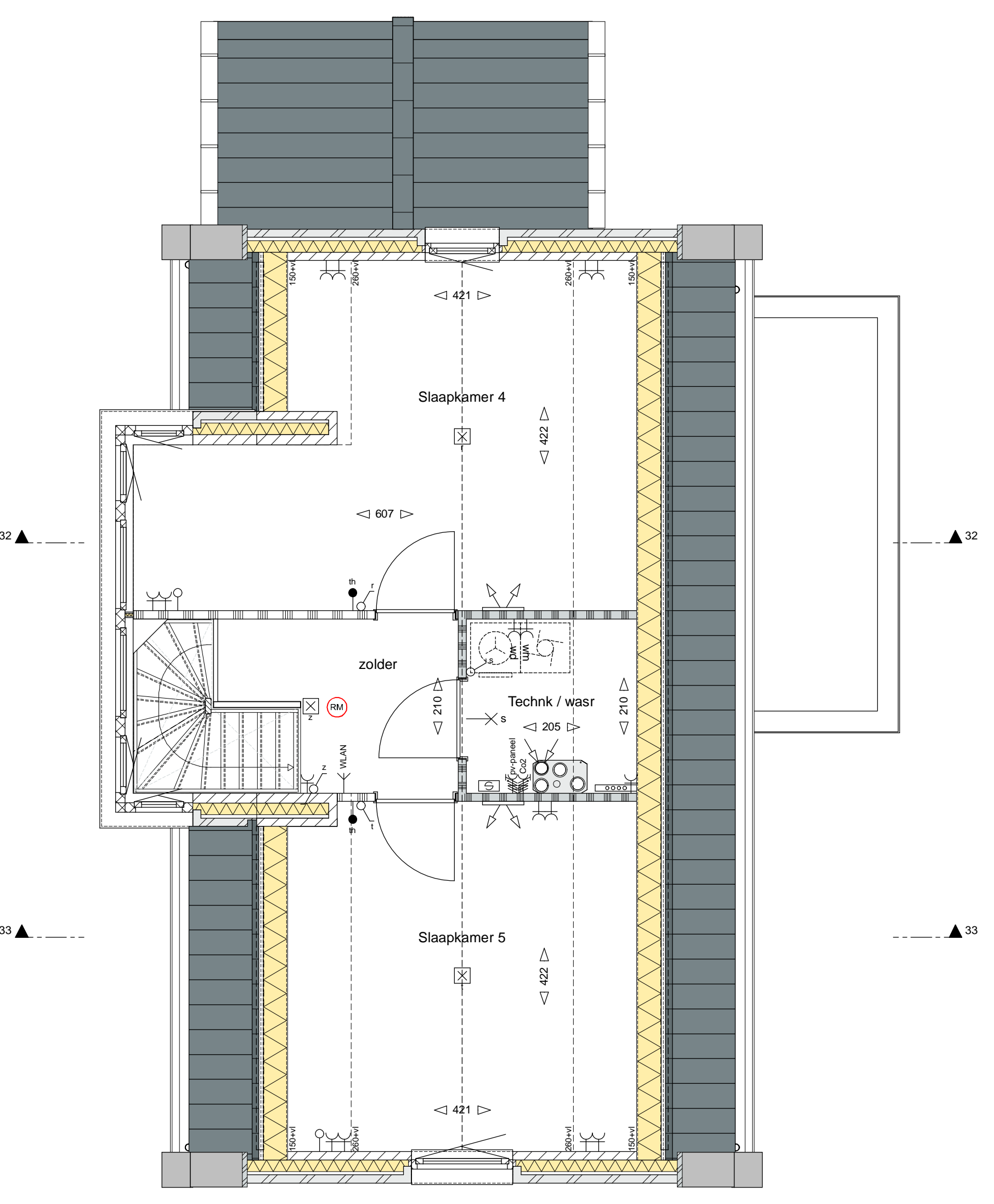
2e verdieping
