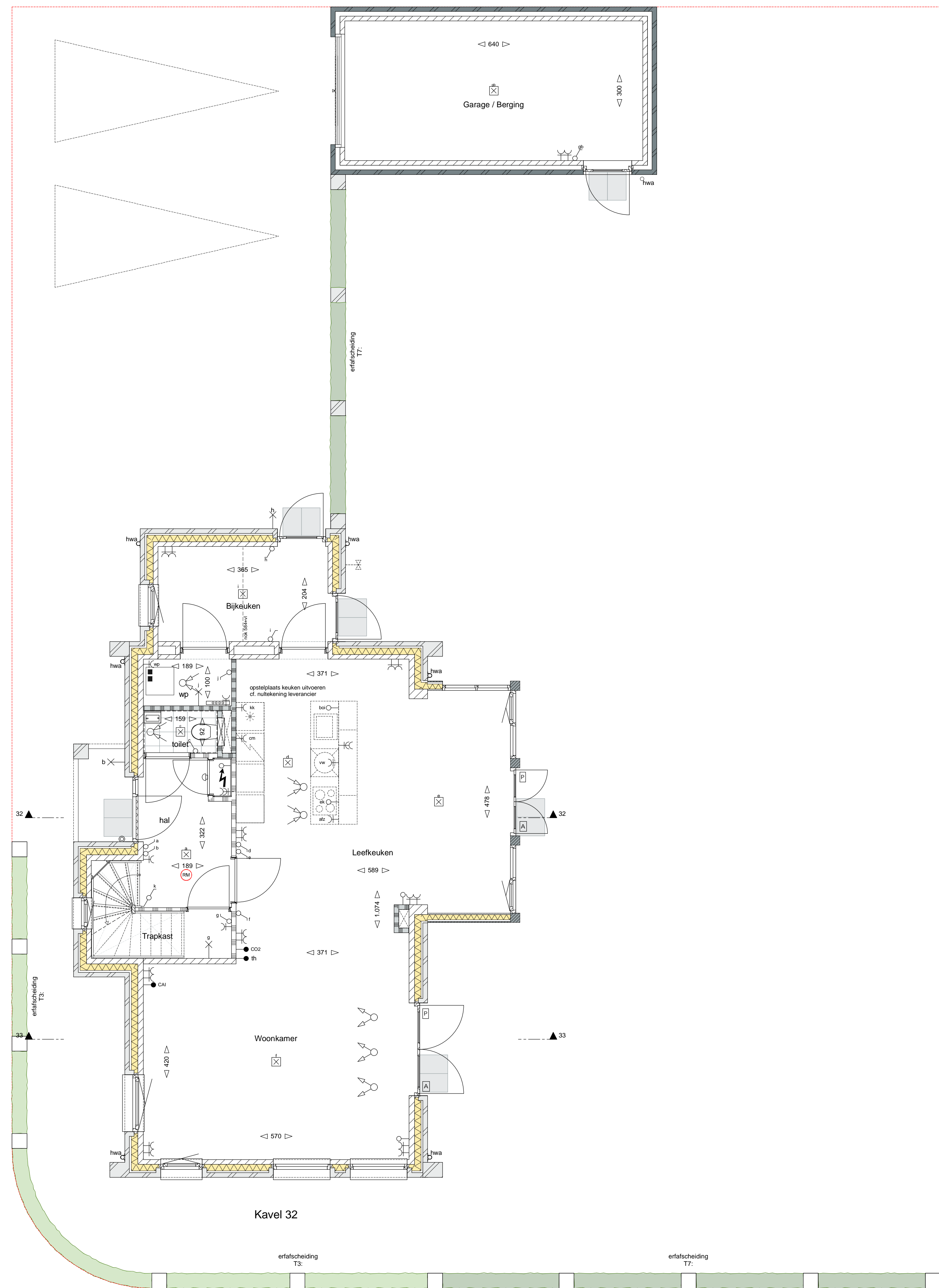
Begane grond
