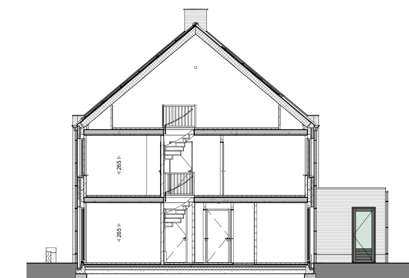
dwarsdoorsnede A-A
