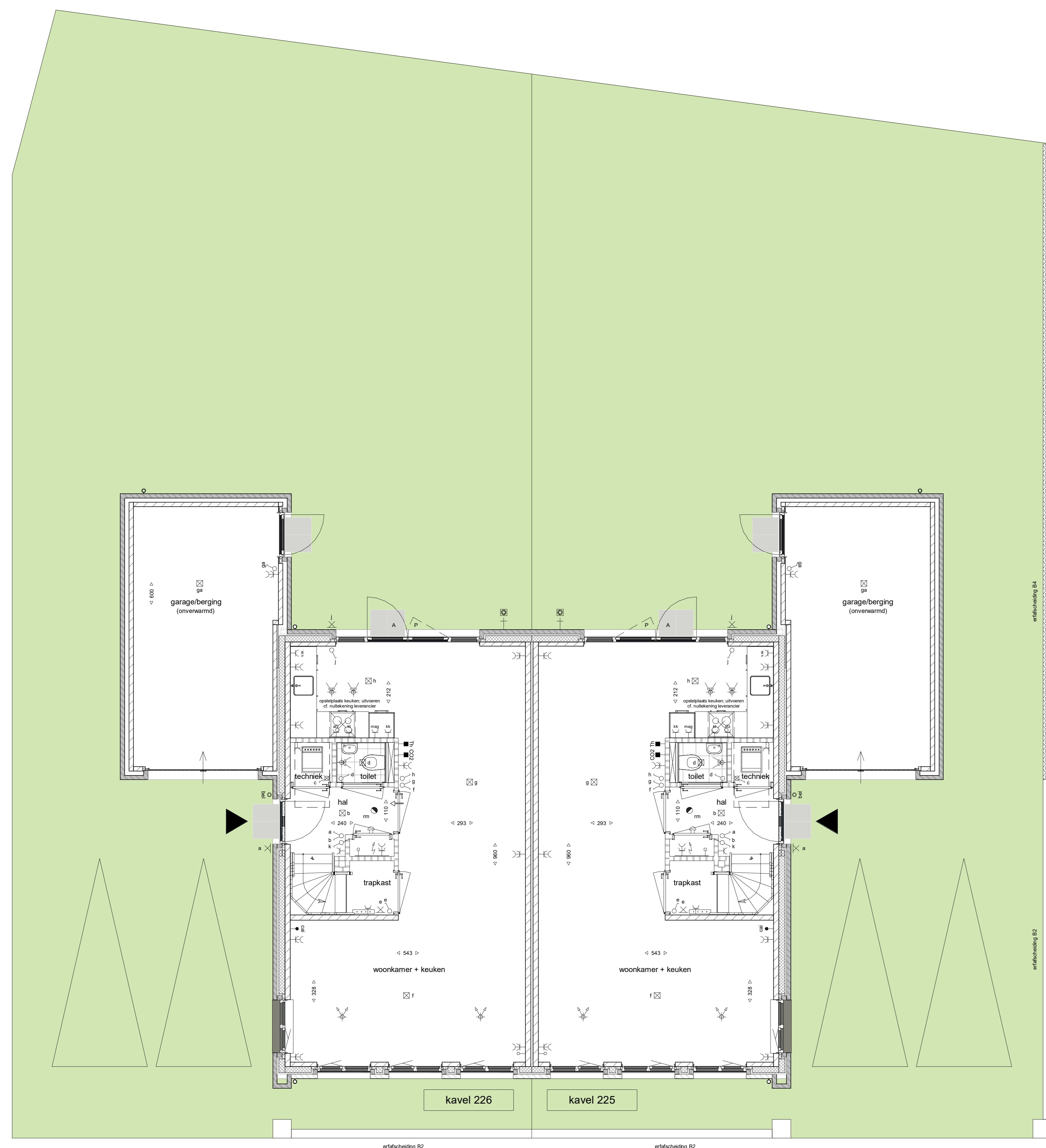
begane grond
