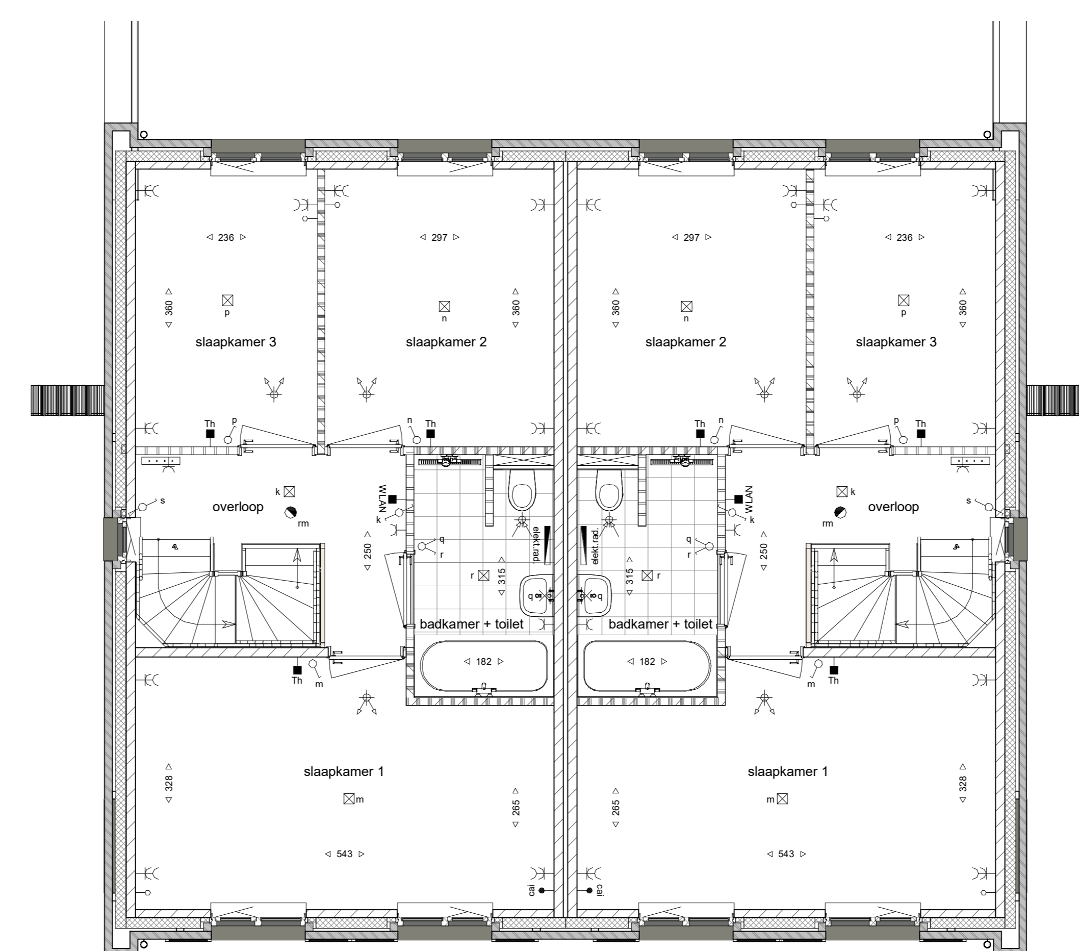
tweede verdieping
