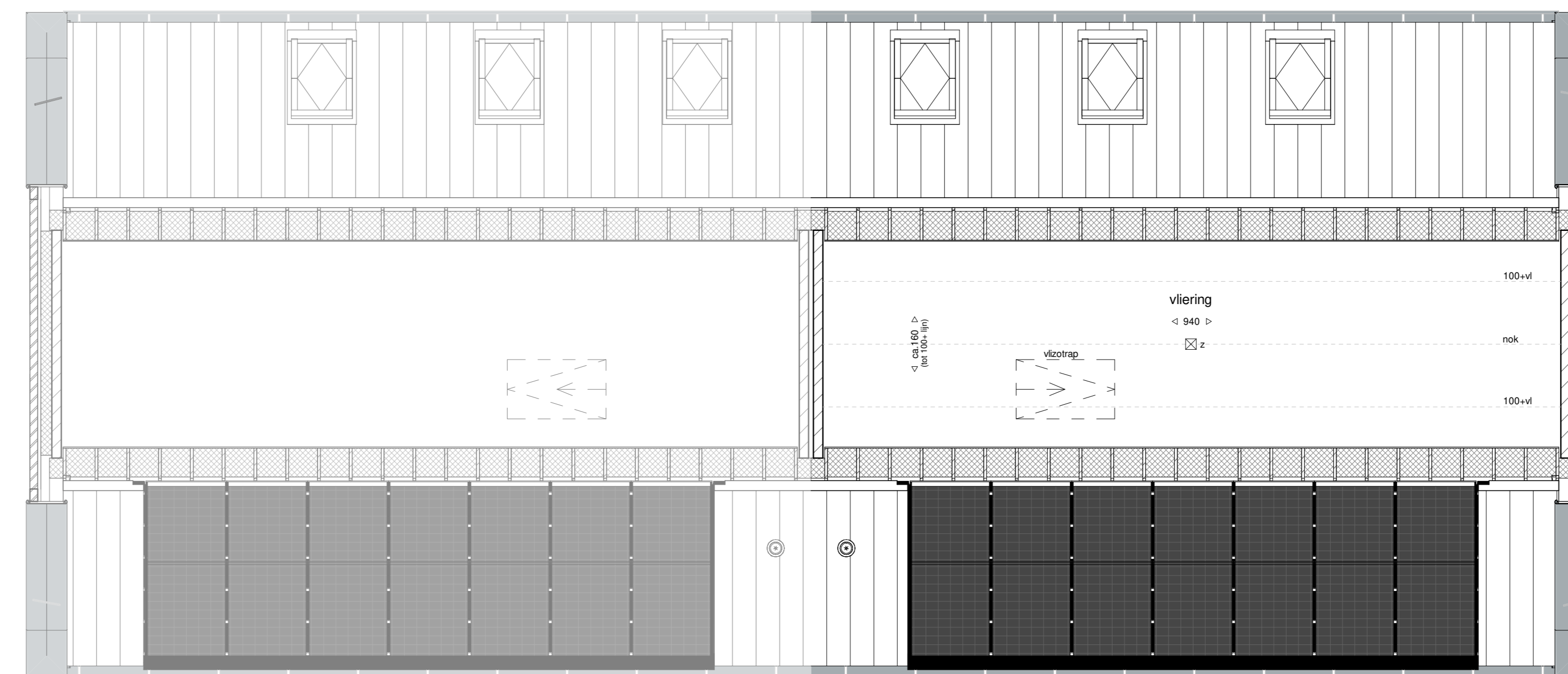
zolder (schaal 1 : 50)
