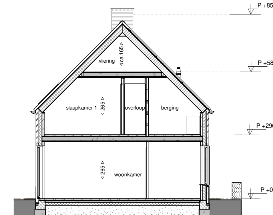
dwarsdoorsnede (schaal 1 : 100)
