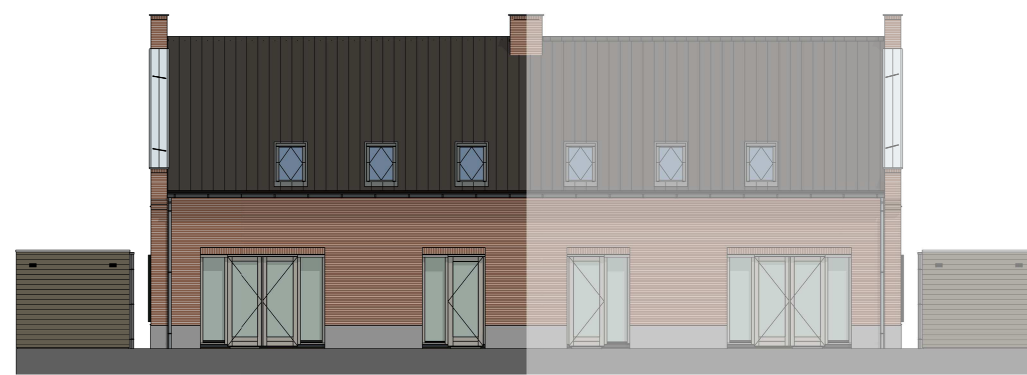
achtergevel (schaal 1 : 100)
