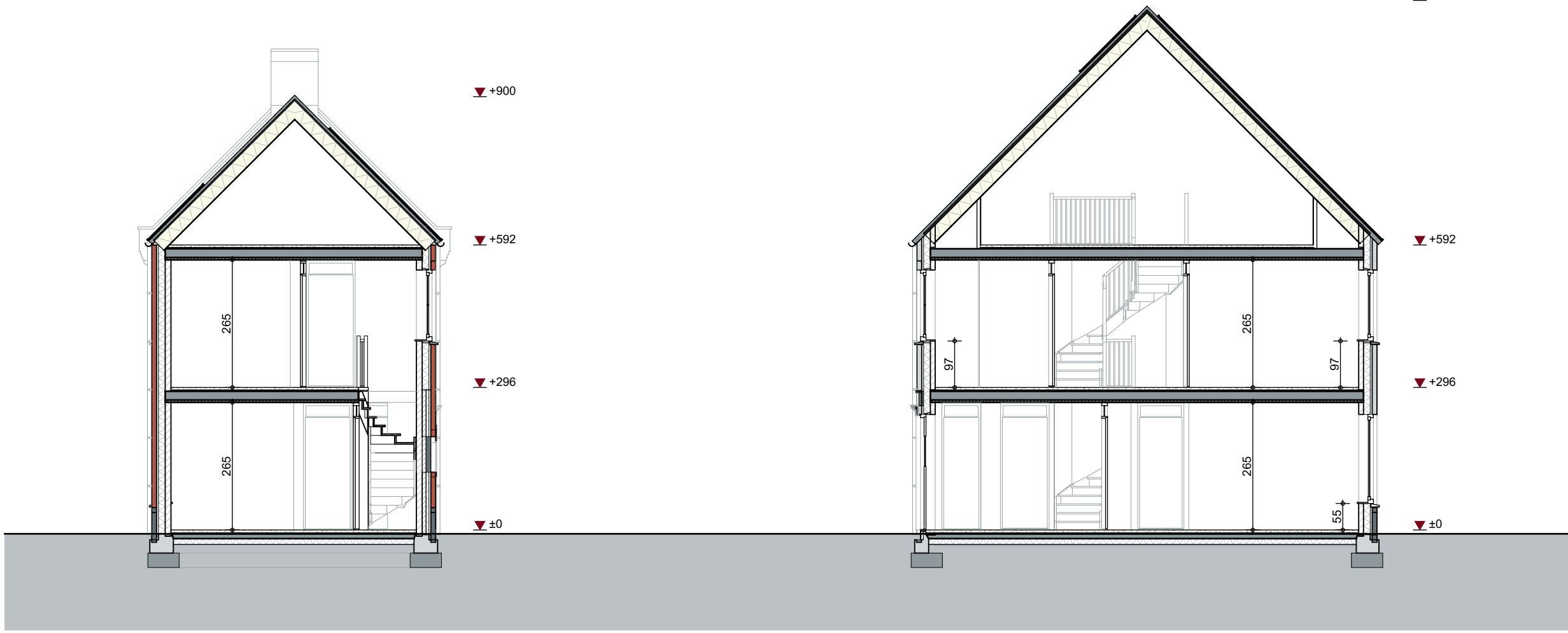
DOORSNEDE 332
