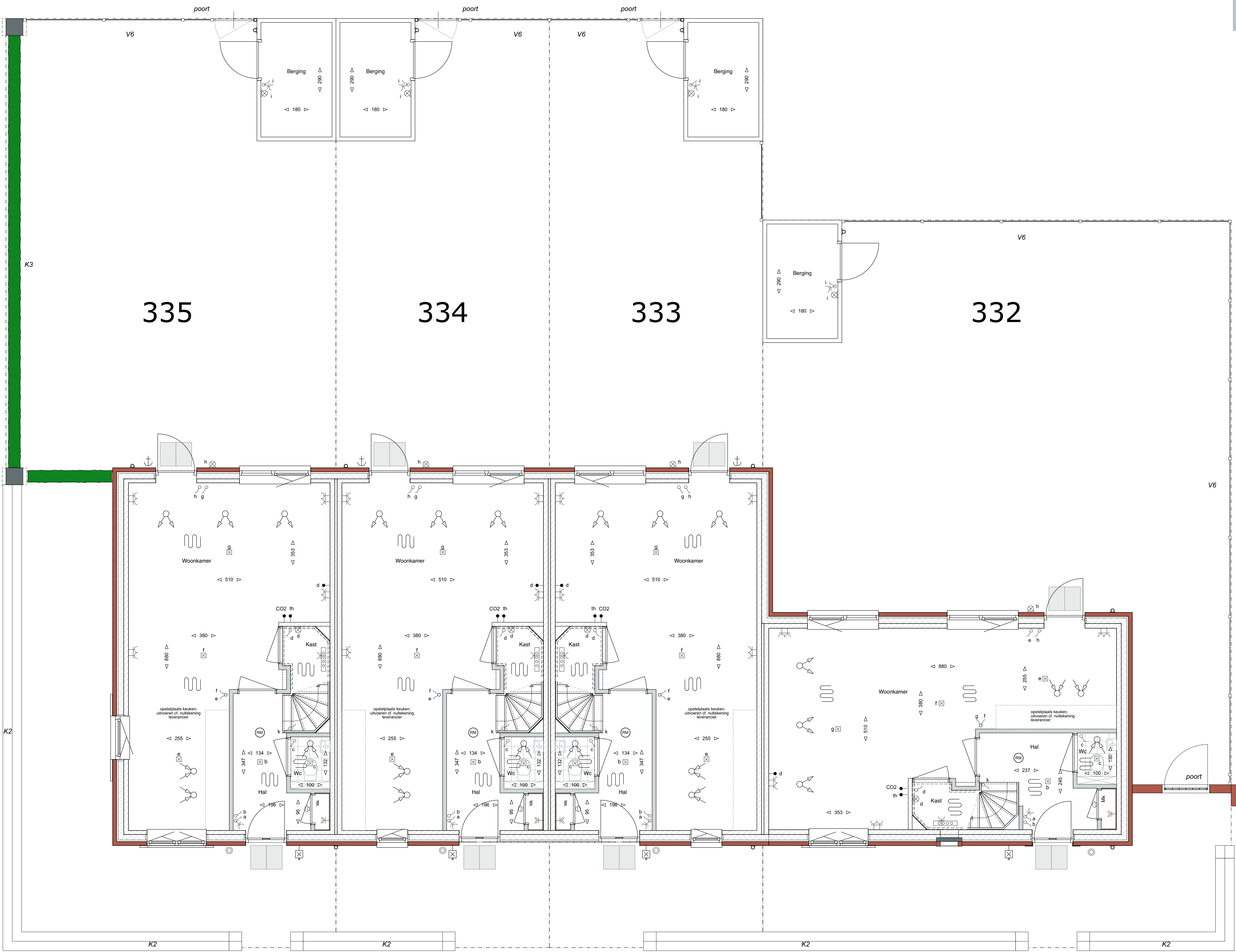
BEGANE GROND
