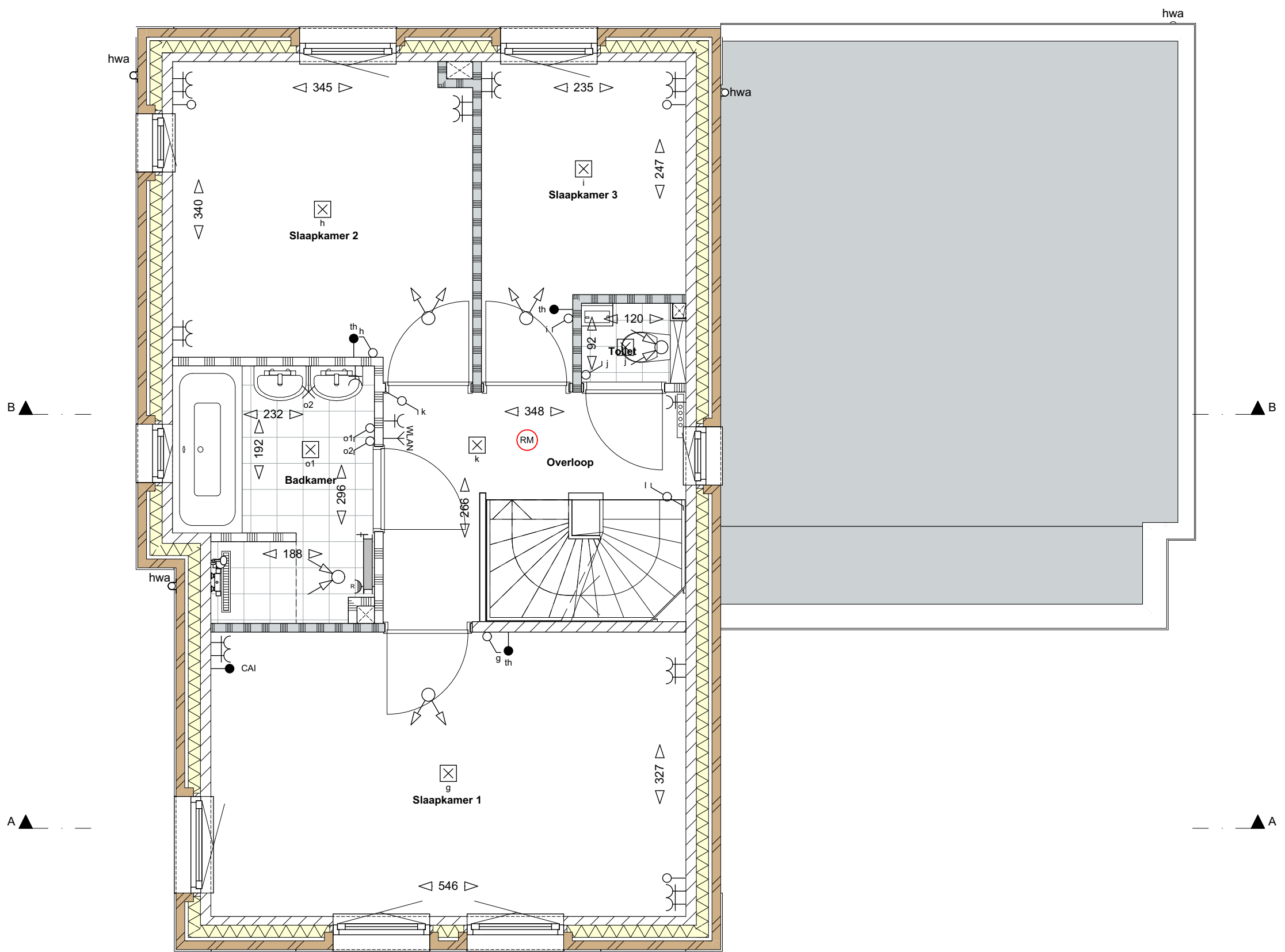
2e verdieping
