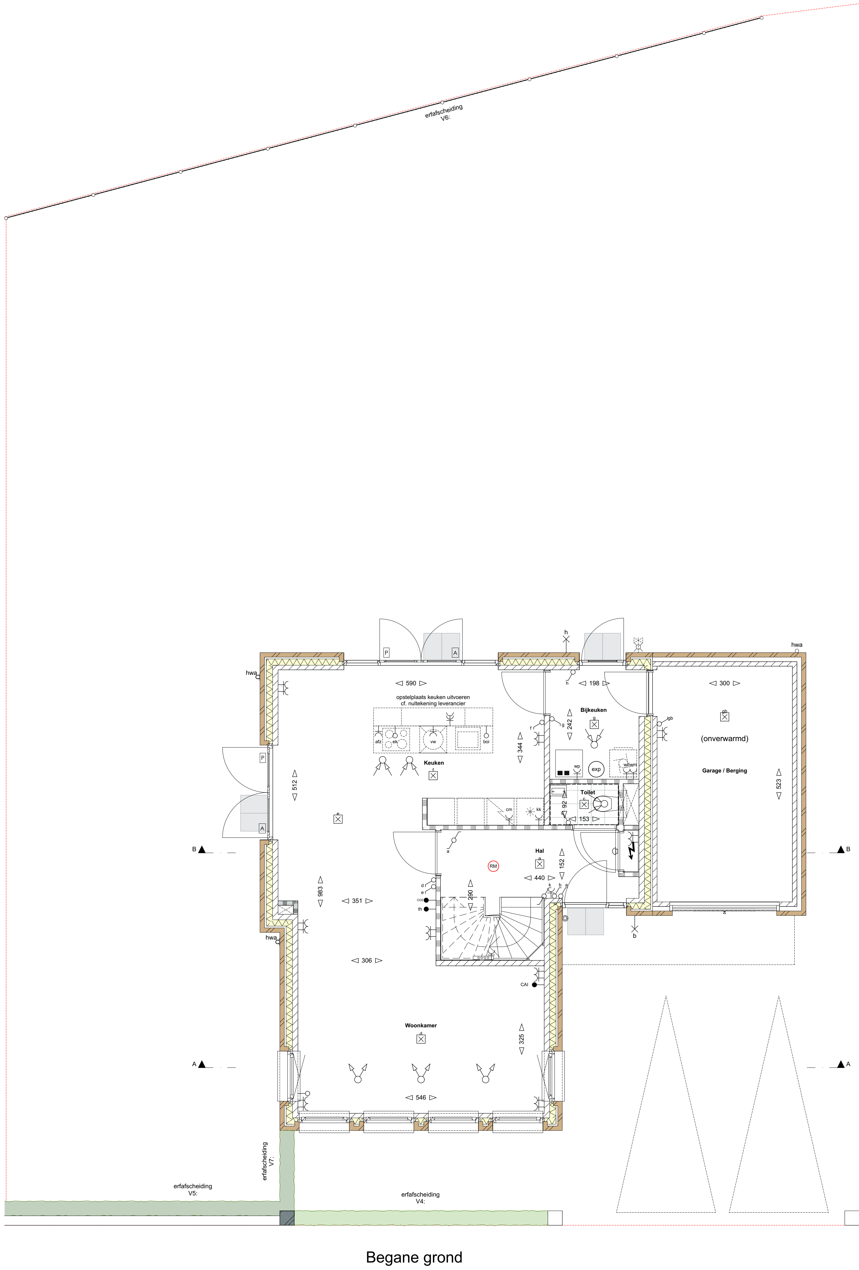
Begane grond
