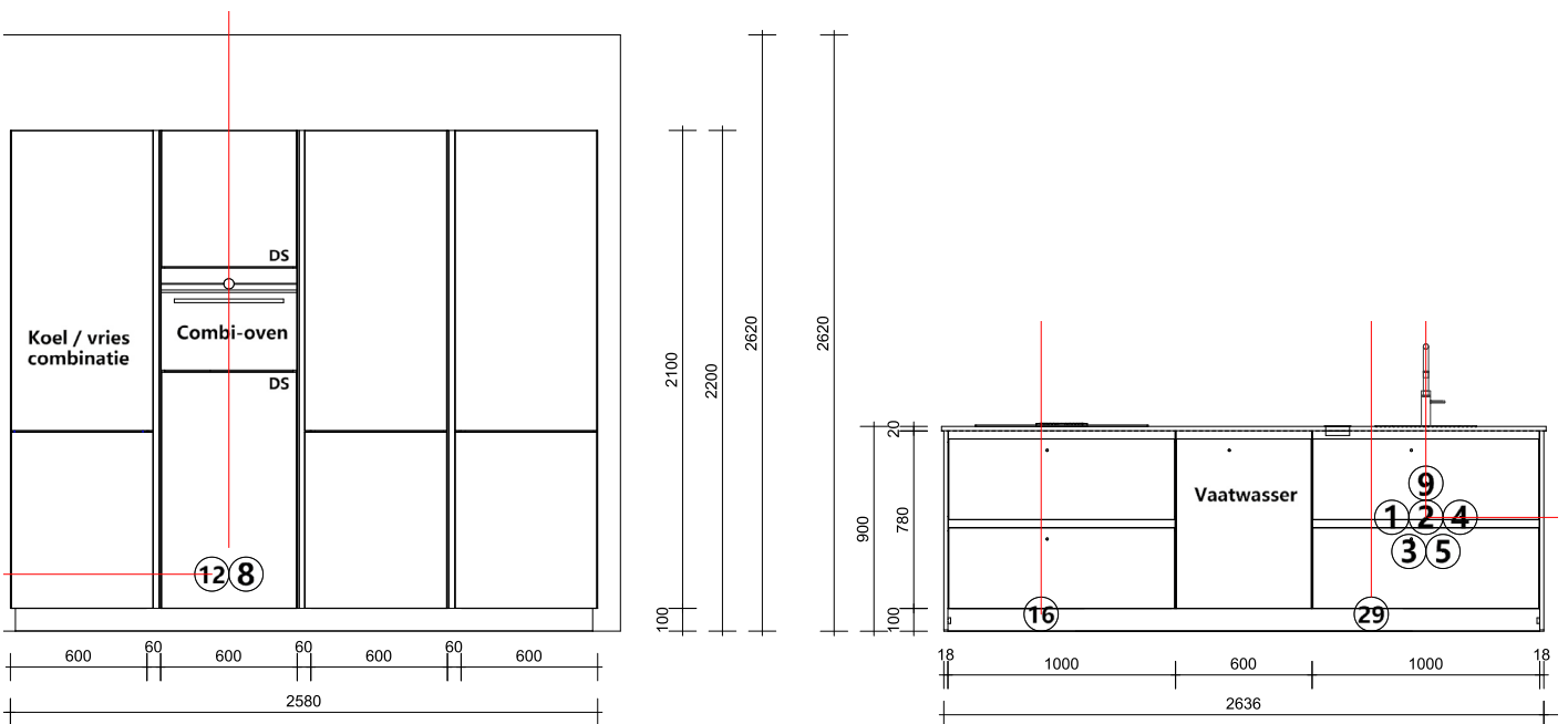
Vooraanzichten
