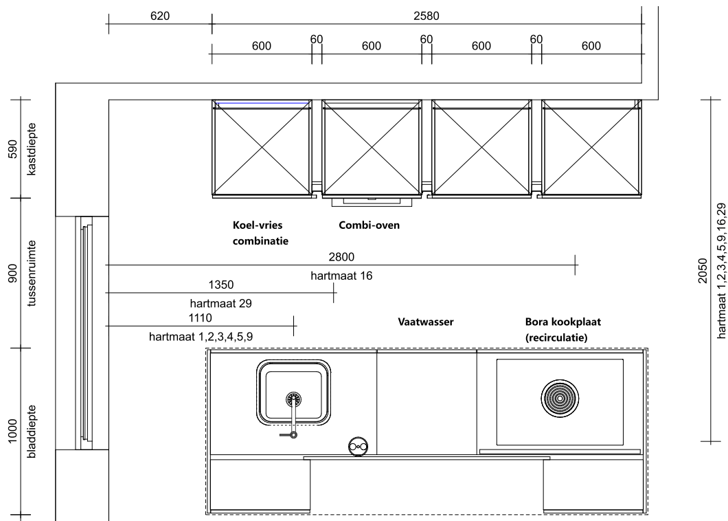
Plattegrond
