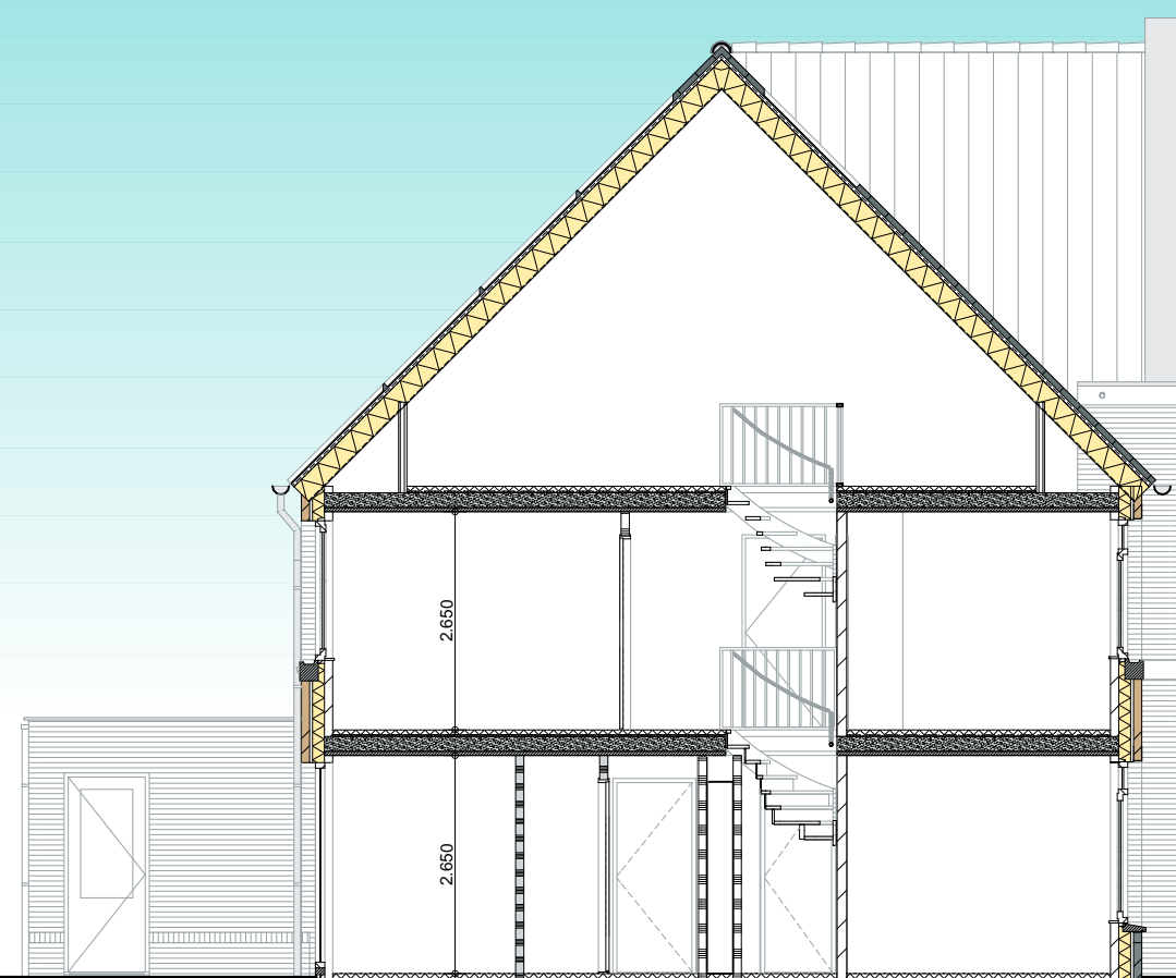
Doorsnede 158
