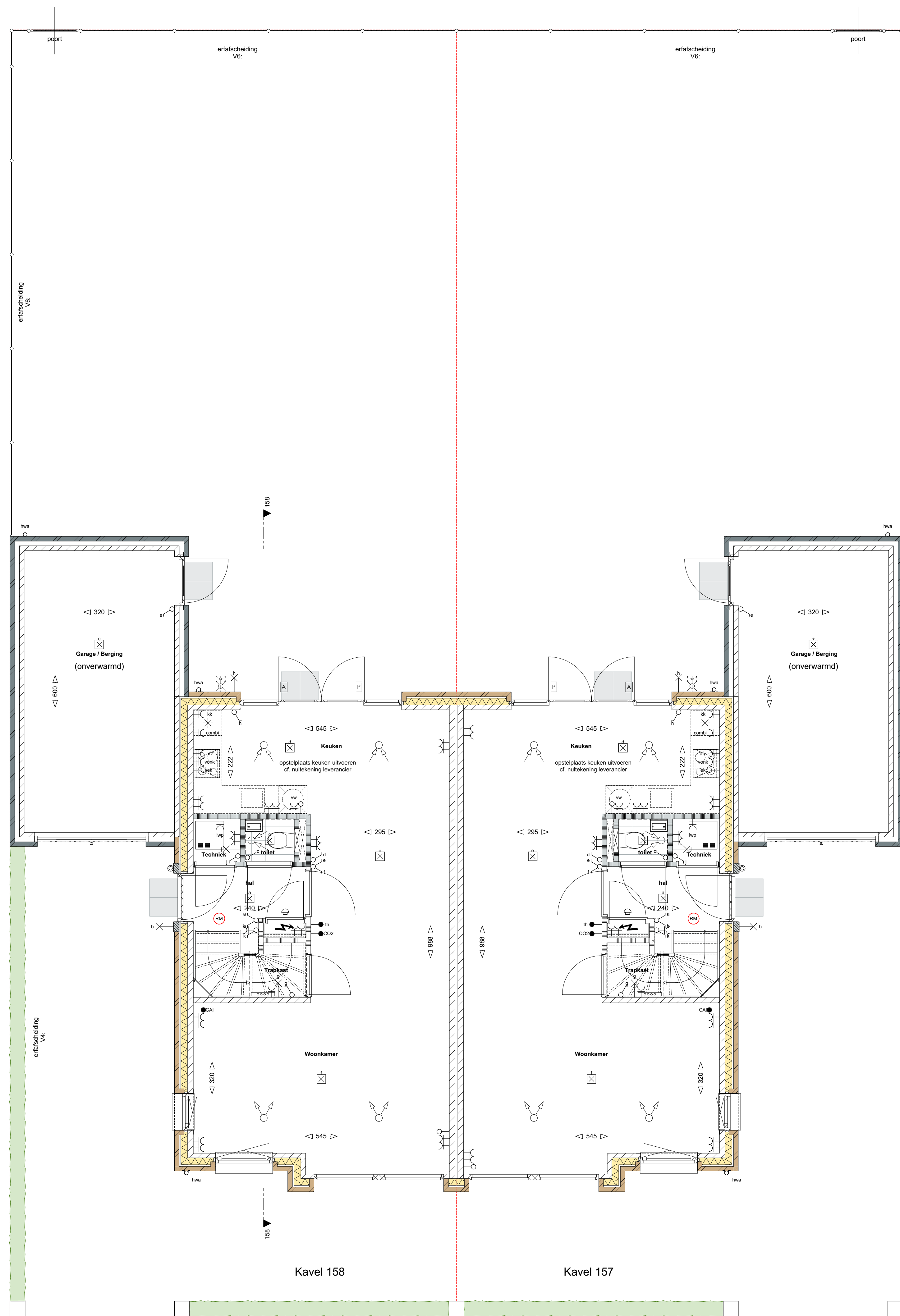
Begane grond
