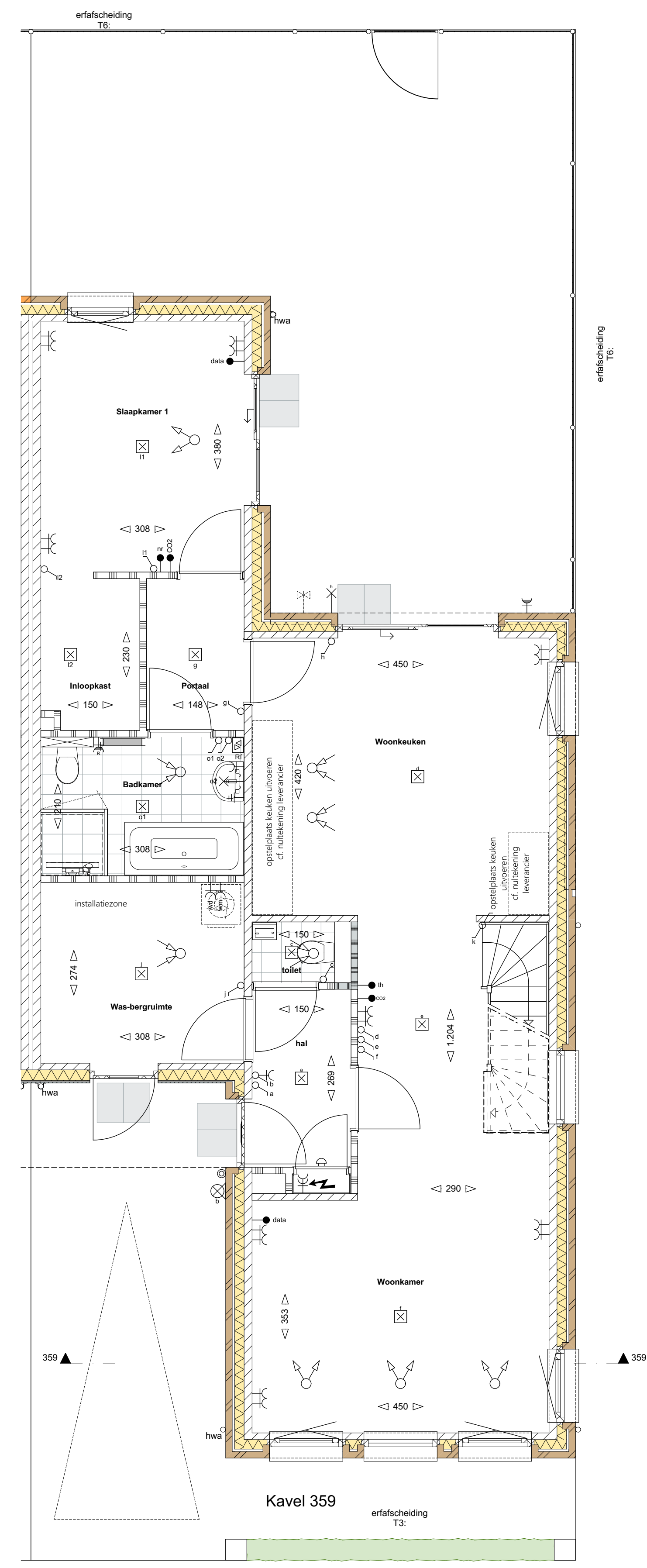
Begane grond
