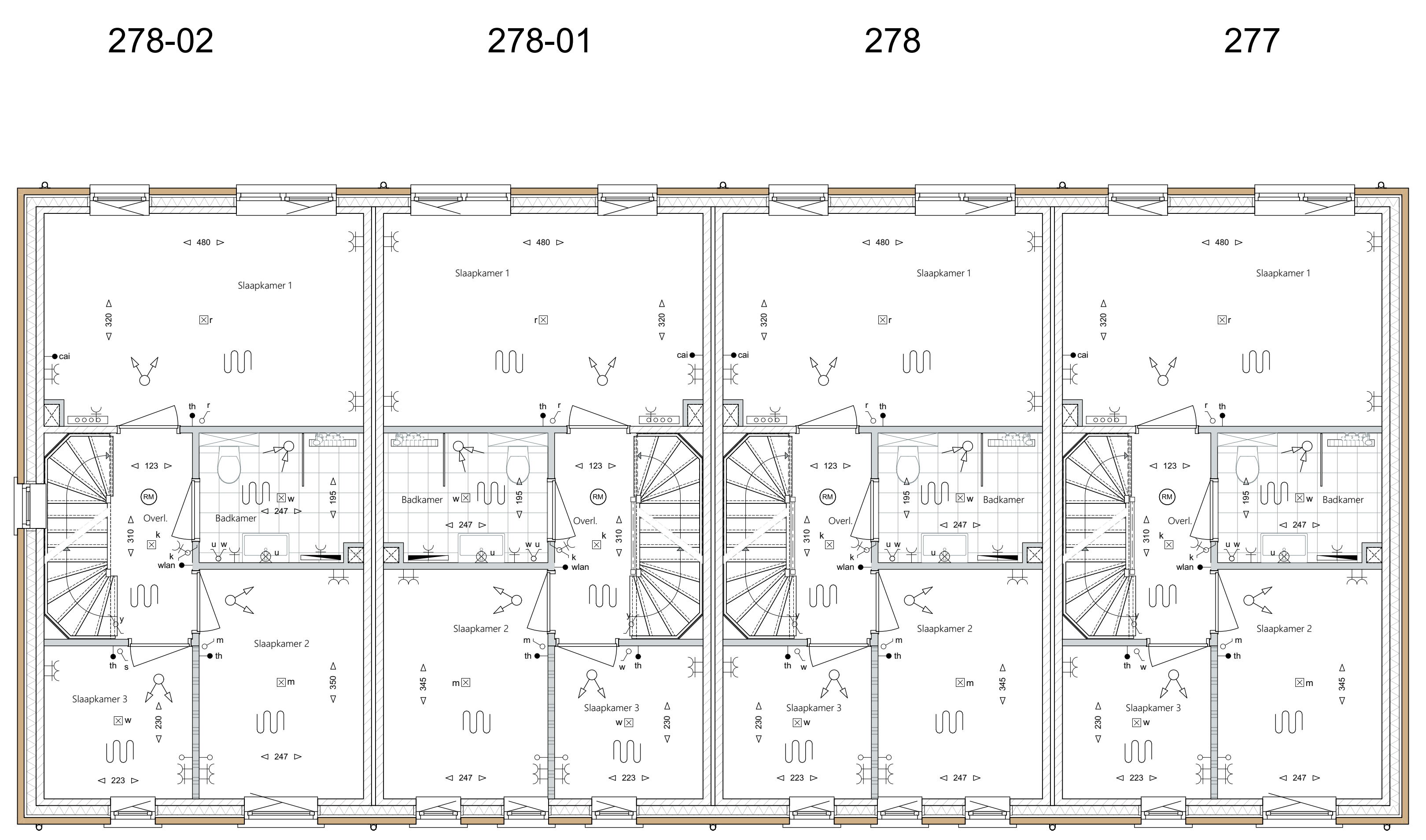
VERDIEPING 2
