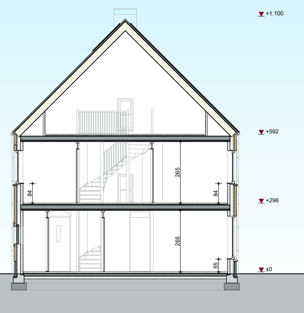
DOORSNEDE
