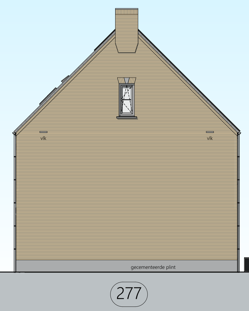
RECHTER ZIJGEVEL
