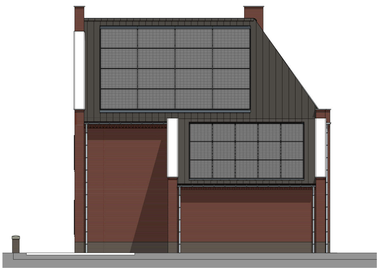
zijgevel rechts
