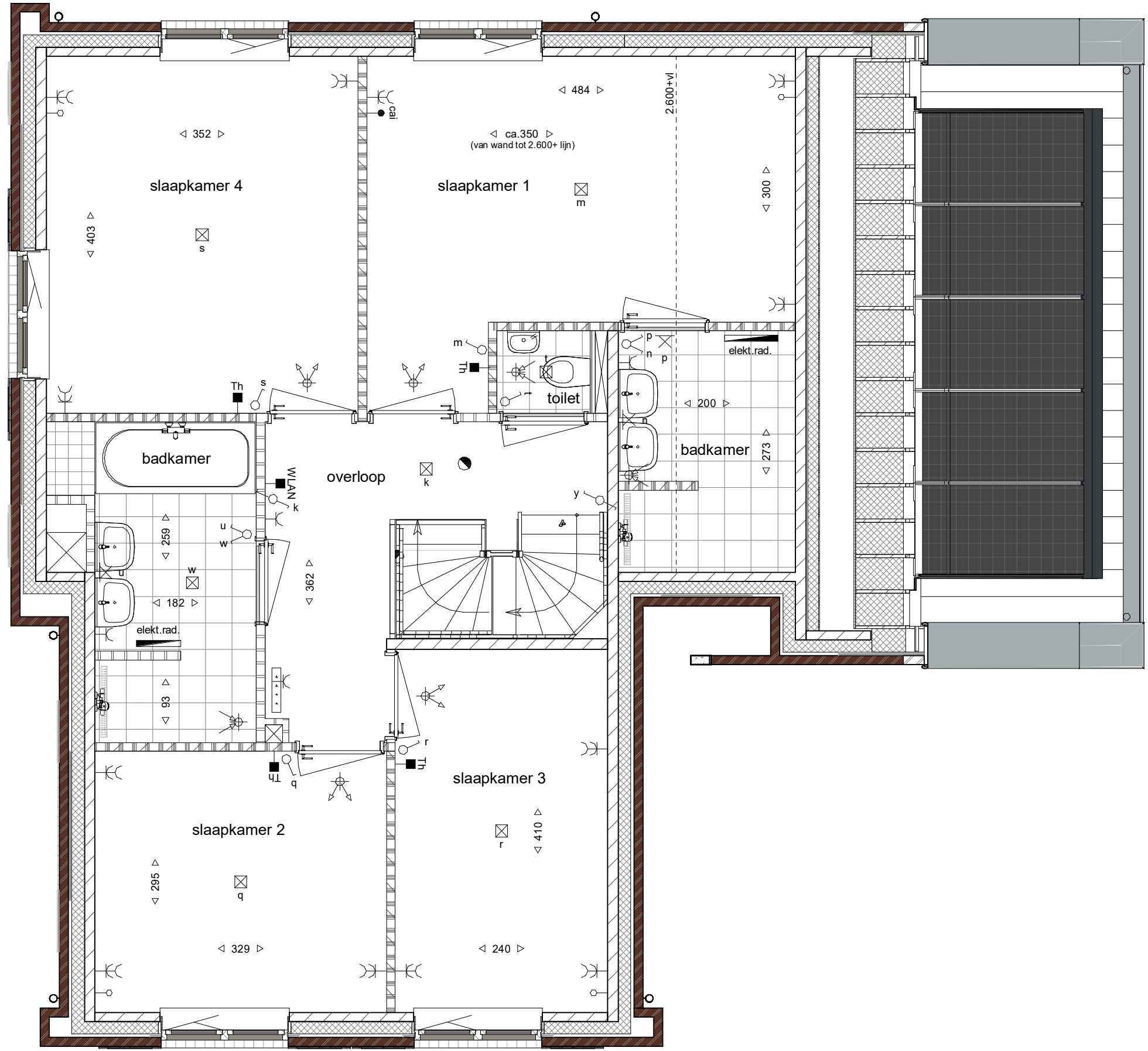
eerste verdieping
