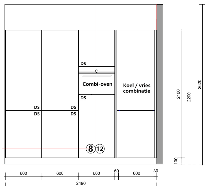
Vooraanzichten
