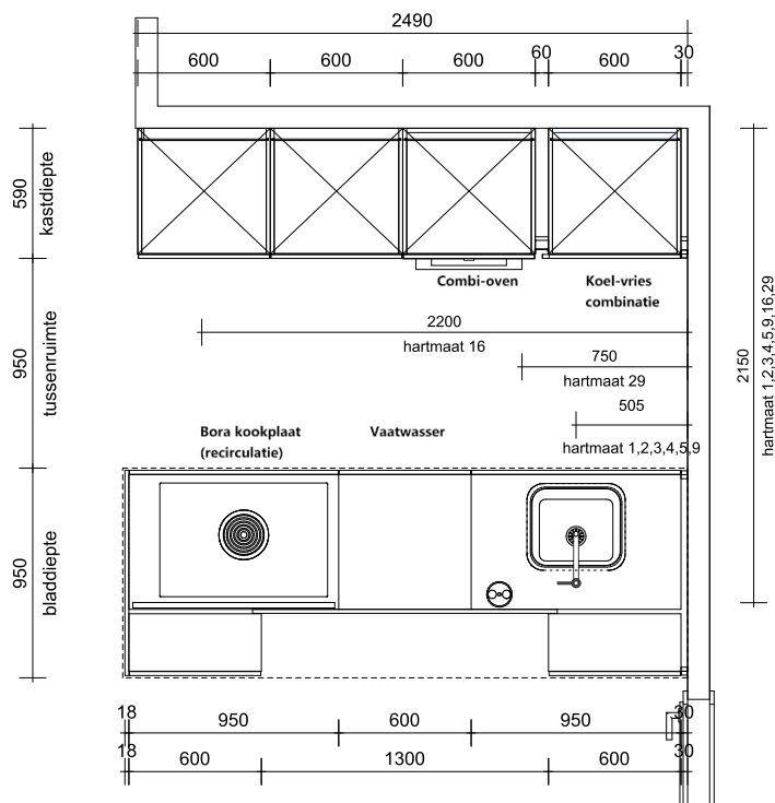
Plattegrond
