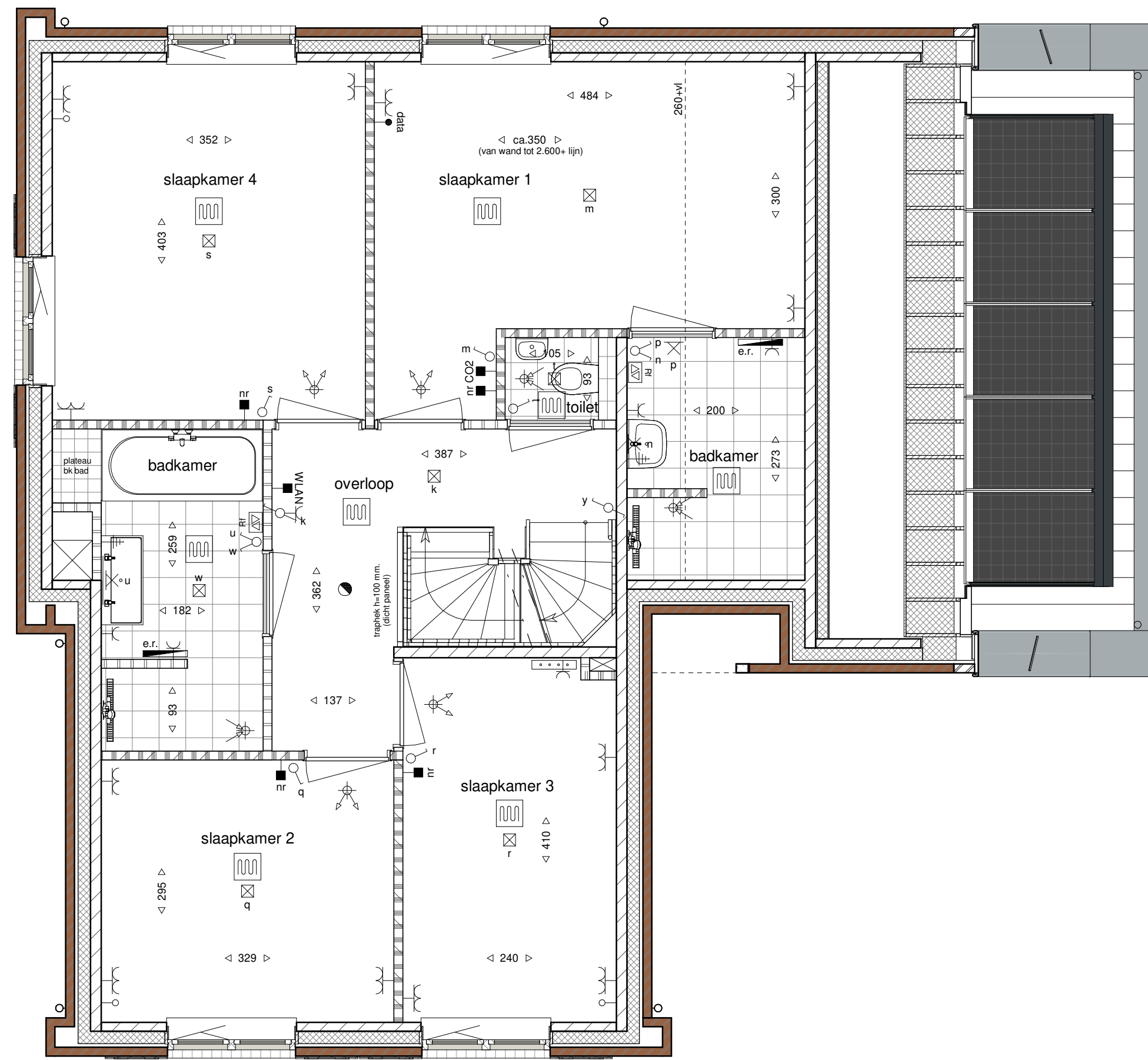
eerste verdieping 1 : 50
