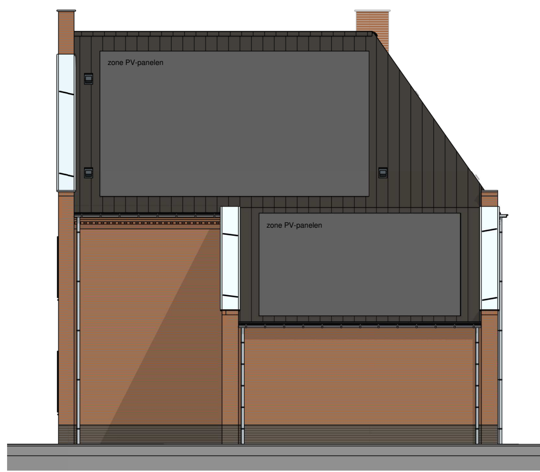
zijgevel rechts 1 : 100
