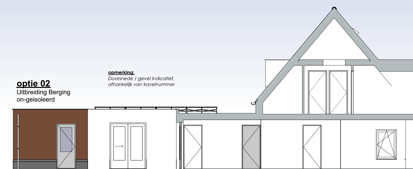
Linkergevel Optie 02
