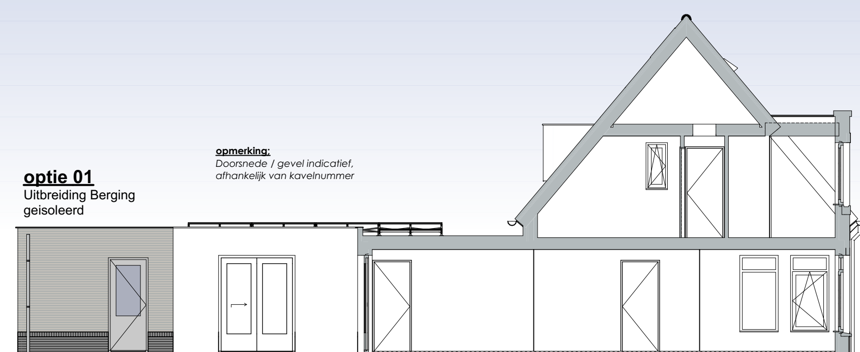
Linkergevel Optie 01
