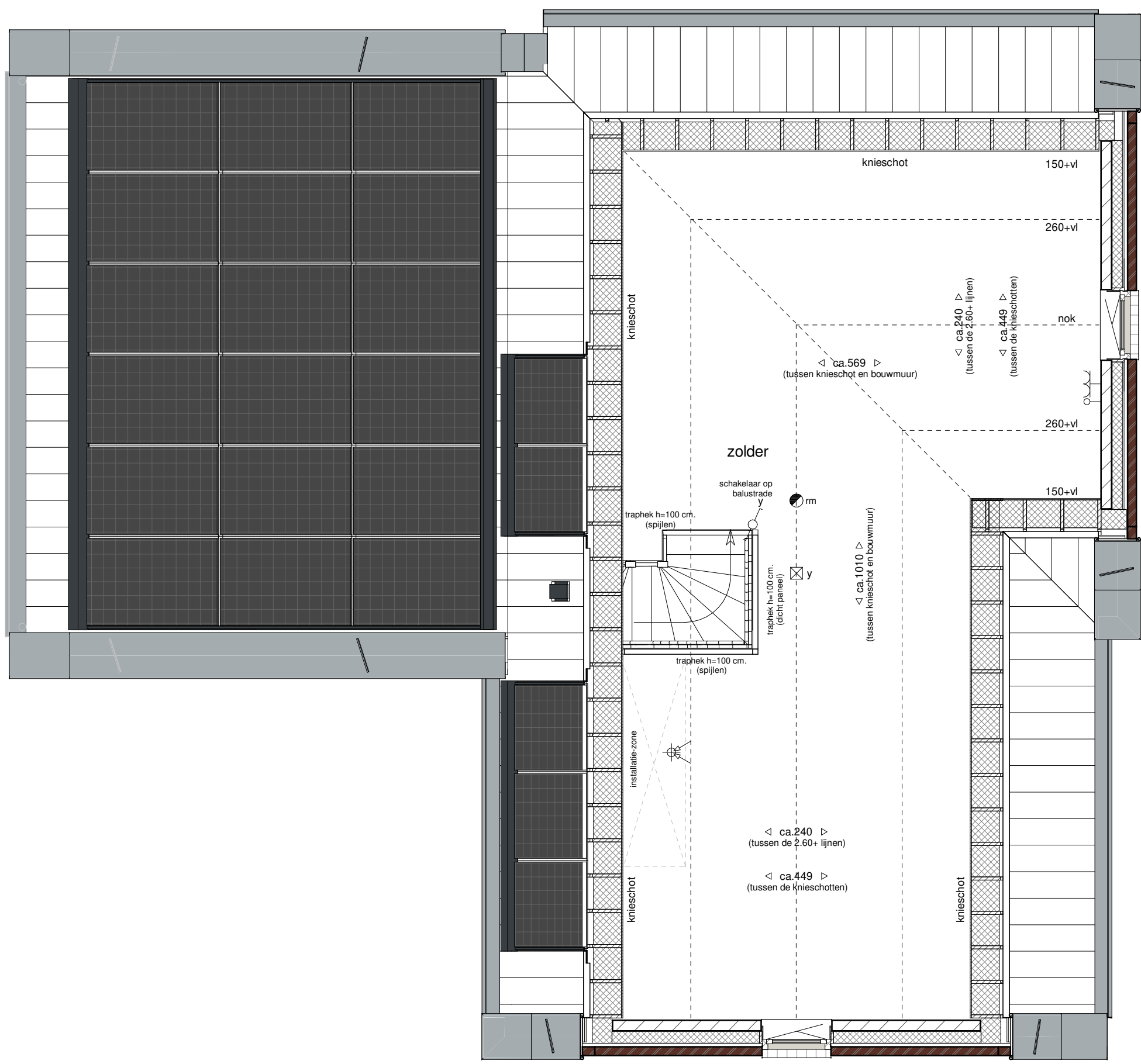
tweede verdieping 1 : 50
