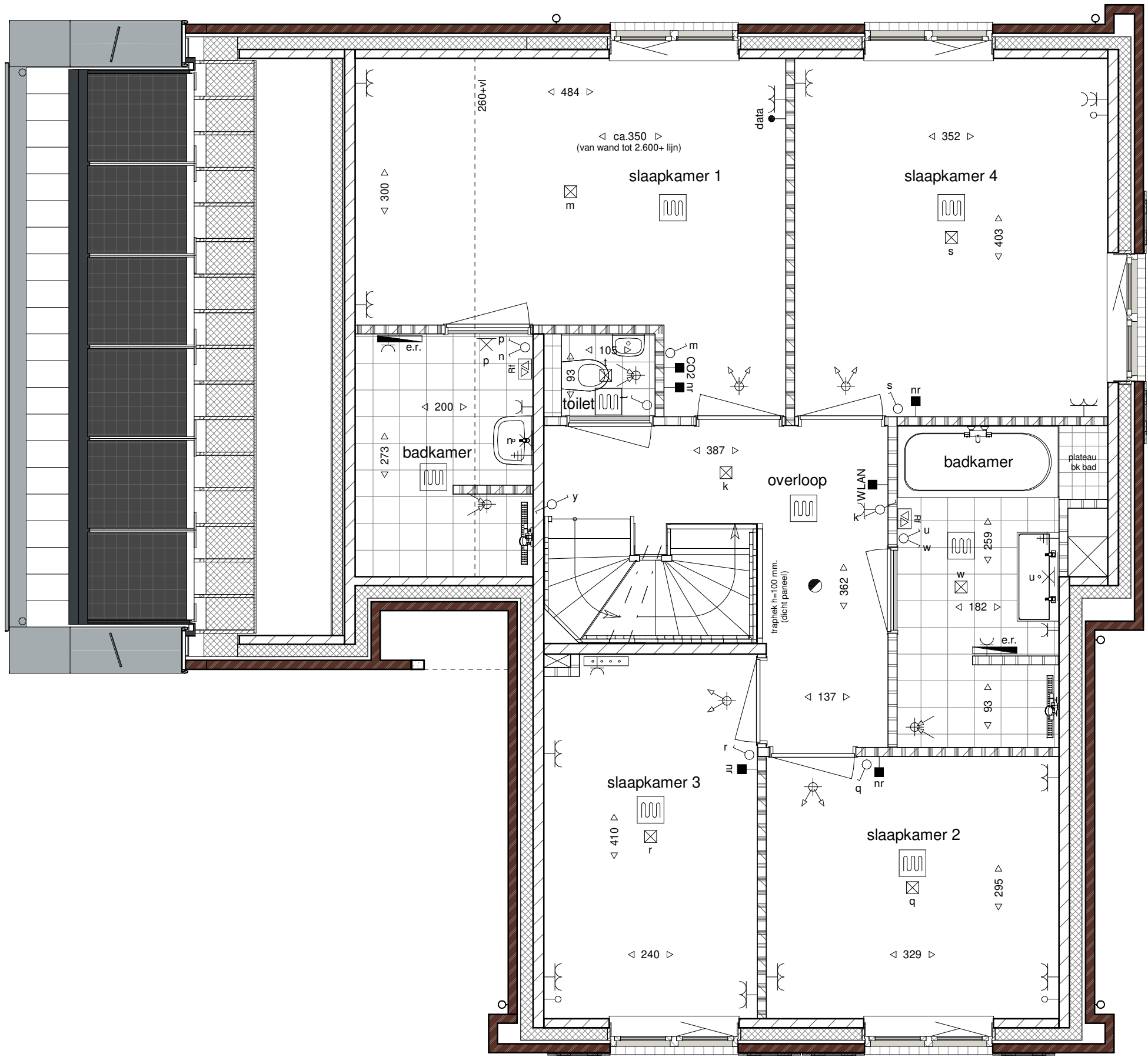
eerste verdieping 1 : 50
