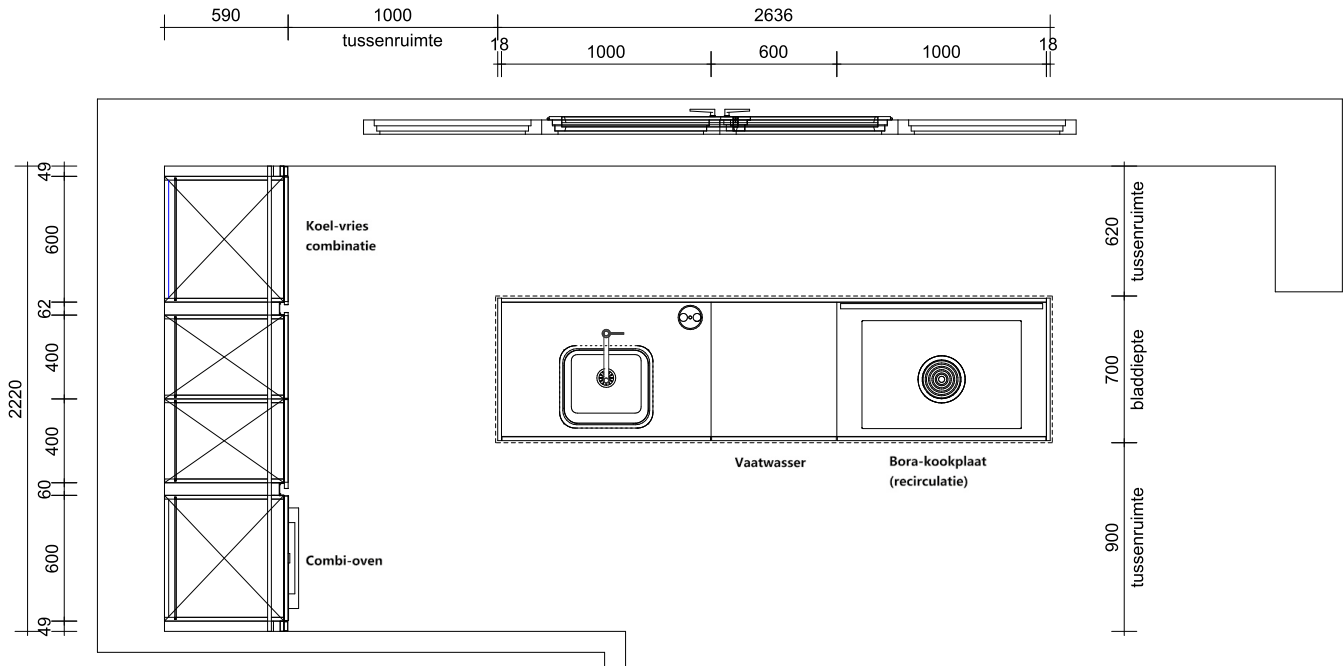
Plattegrond
