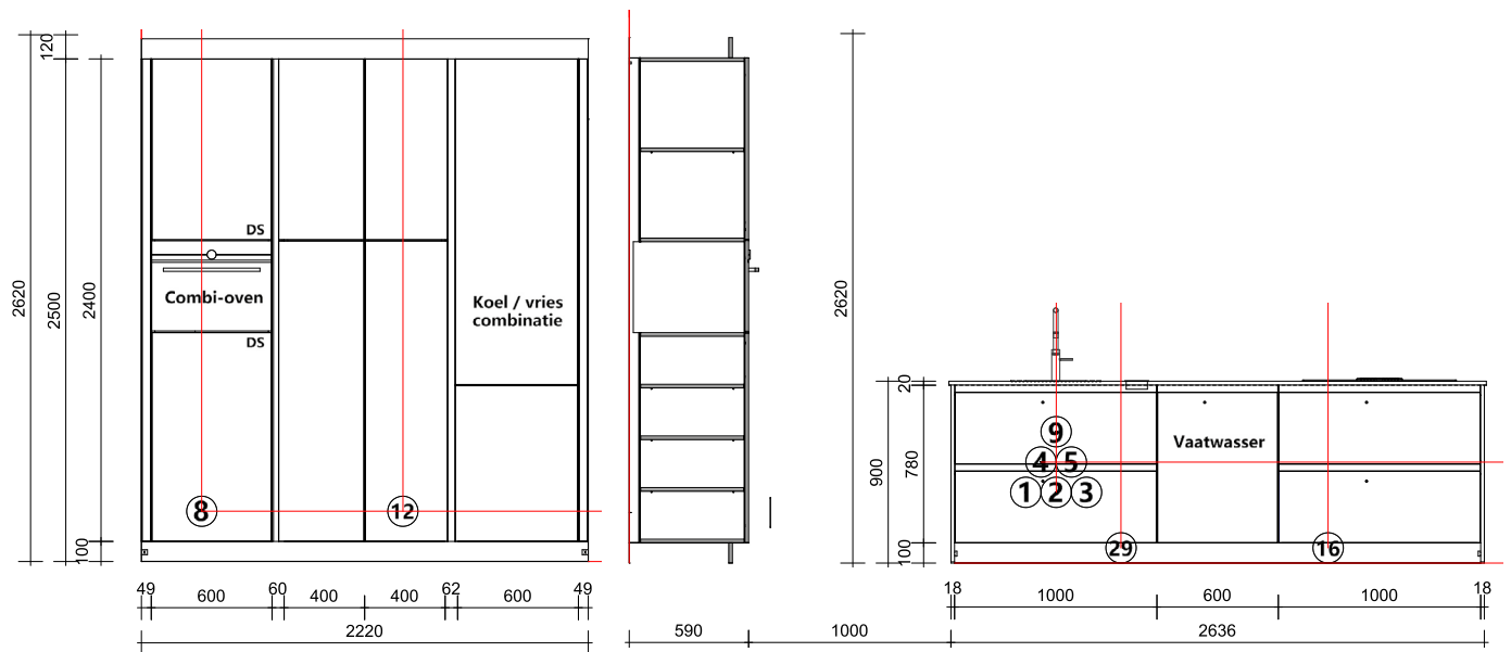
Vooraanzichten
