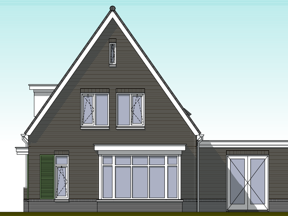
Rechtergevel
