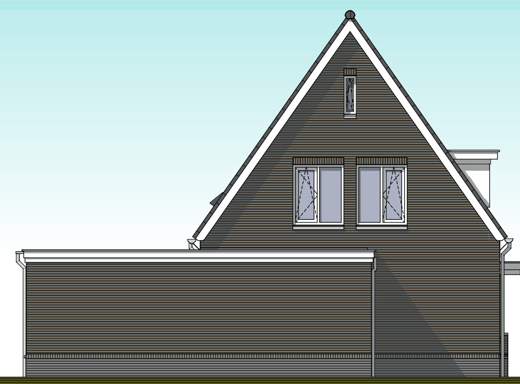
Linkergevel
