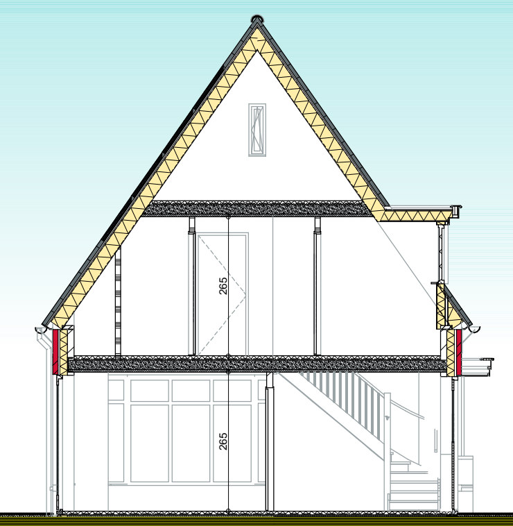
70 Doorsnede 70
