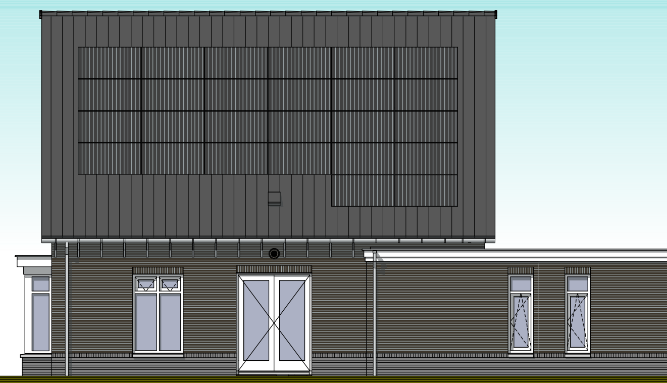
Achtergevel
