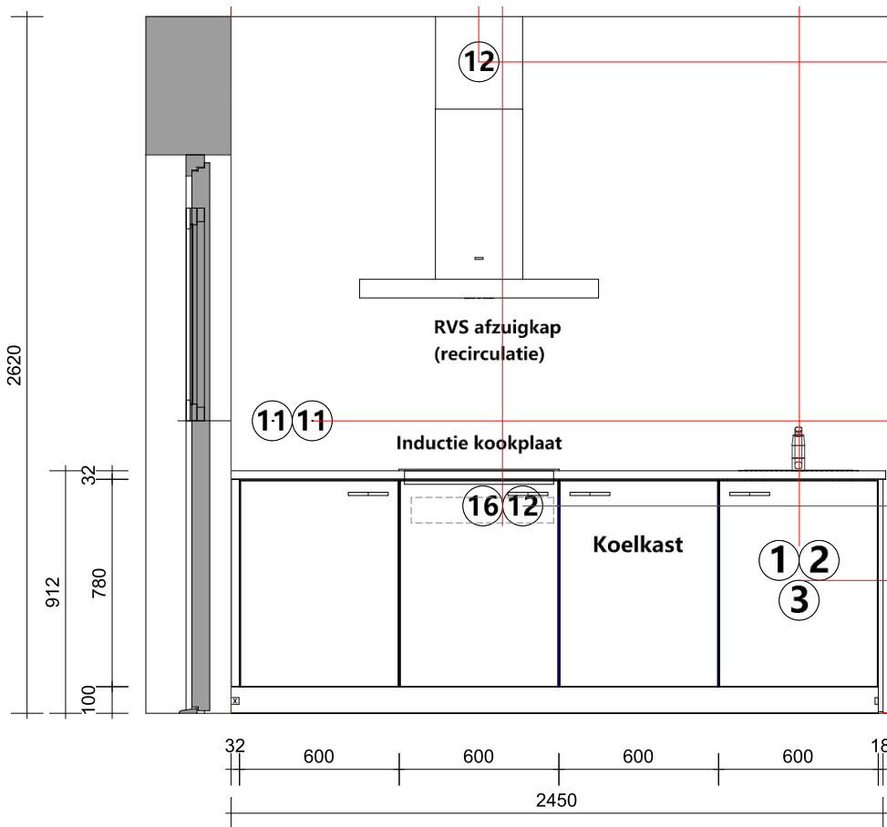
Vooraanzicht
