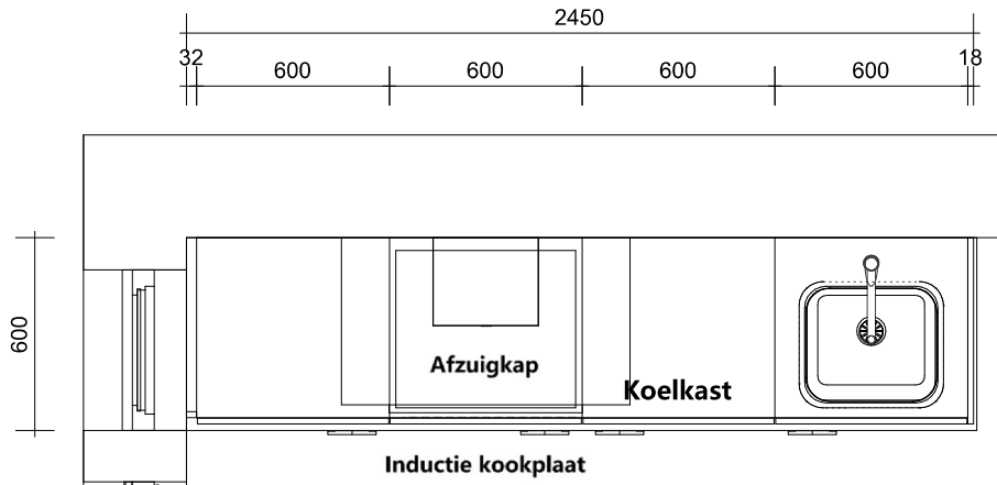
Plattegrond
