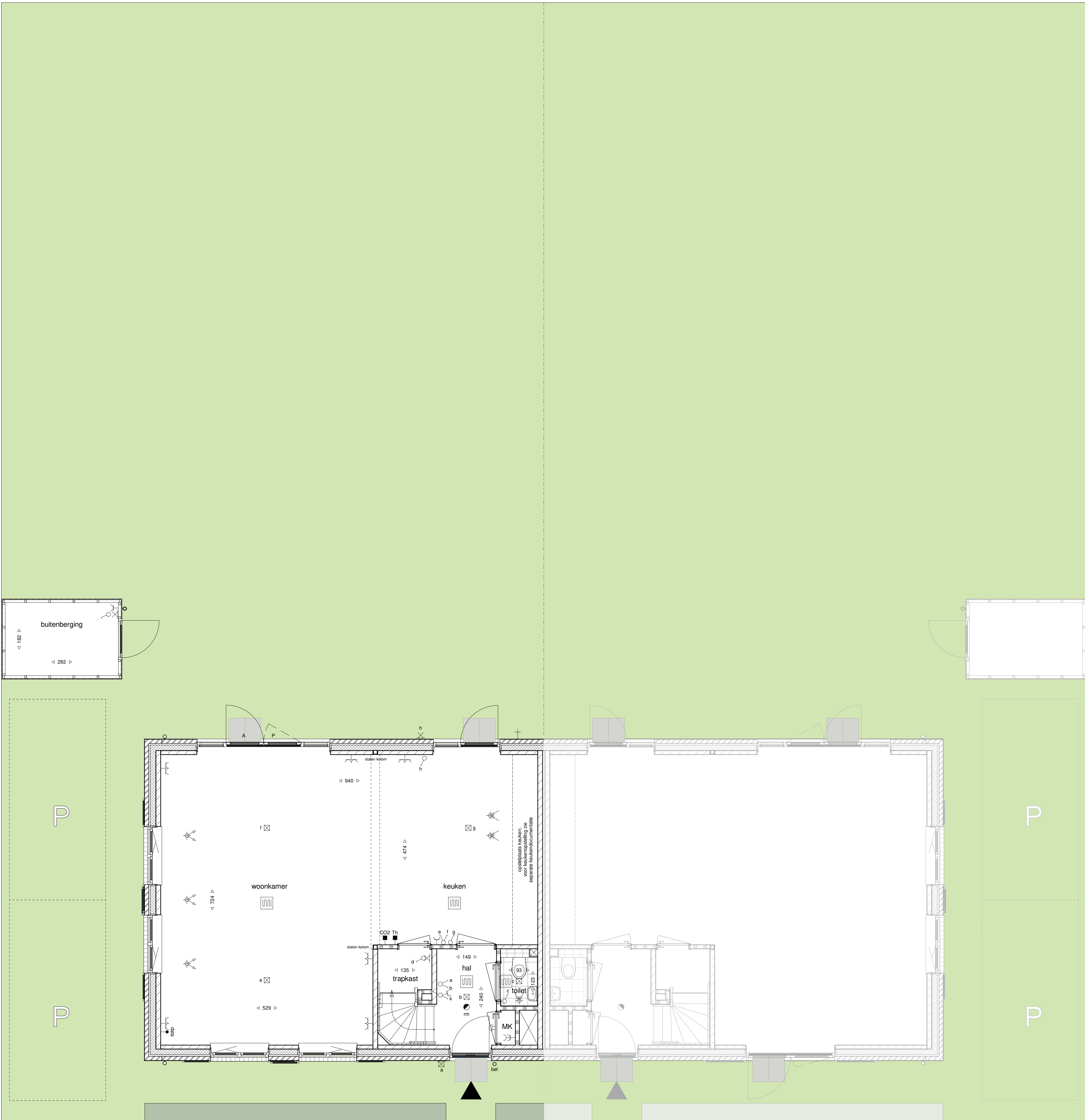
begane grond (schaal 1 : 50)
