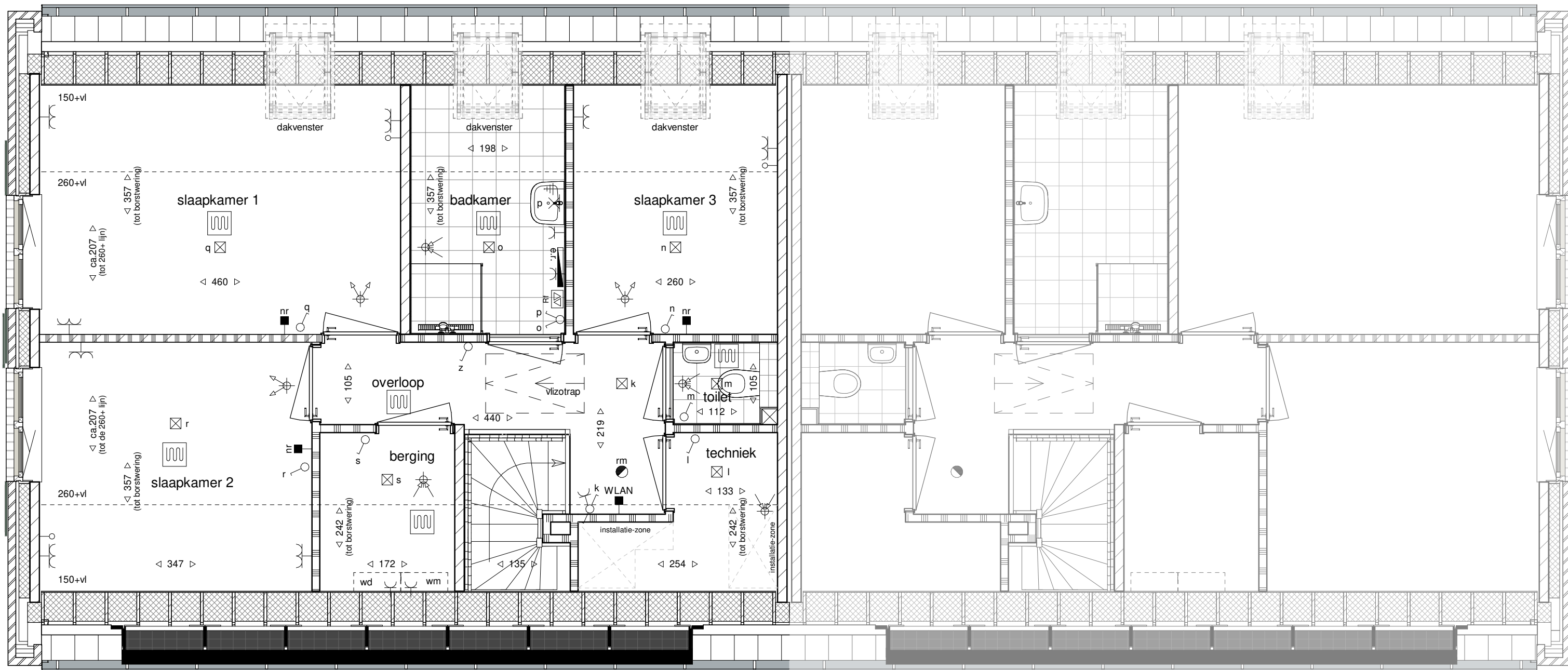
eerste verdieping (schaal 1 : 50)
