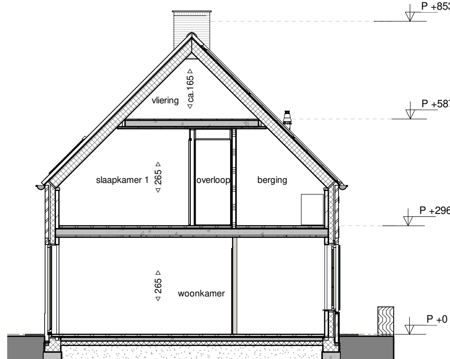
dwarsdoorsnede (schaal 1 : 100)
